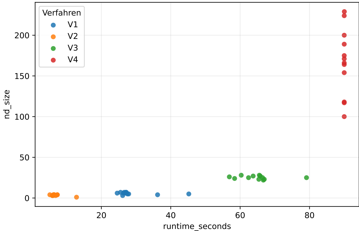
Qualität vs Zeit (medium, schwer)
