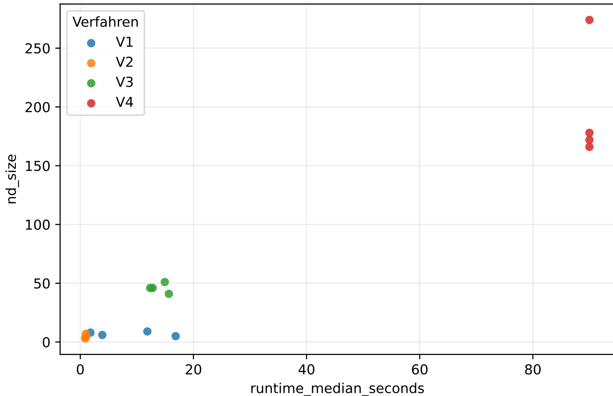
Qualität vs Zeit (small, mittel)
