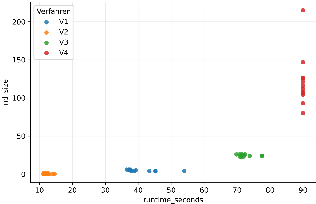
Qualität vs Zeit (large, schwer)
