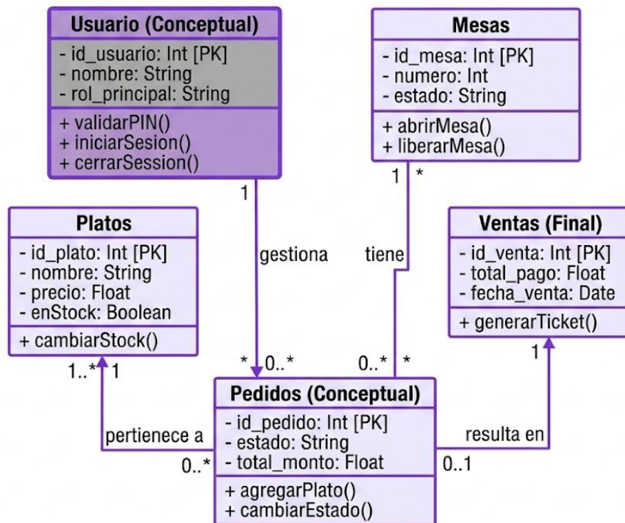
Ejemplo: Diagrama de Clases
