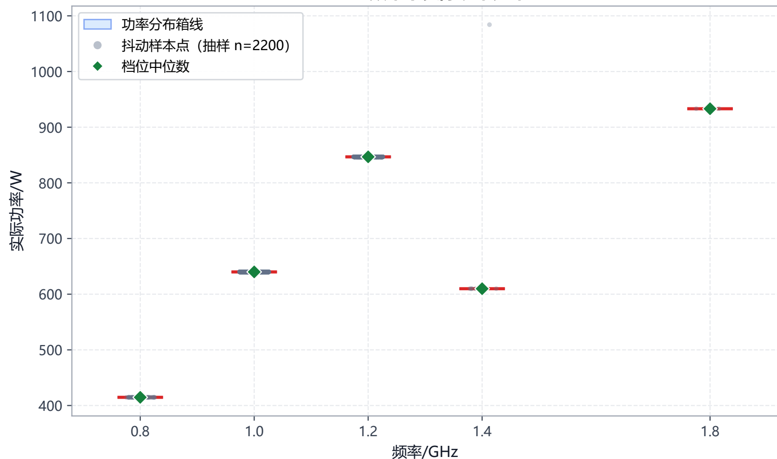
DVFS频率下实际功率分布
