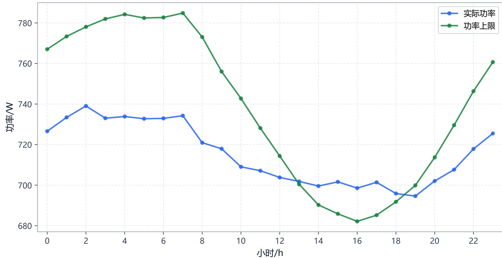
芯片实际功率与功率上限对比
