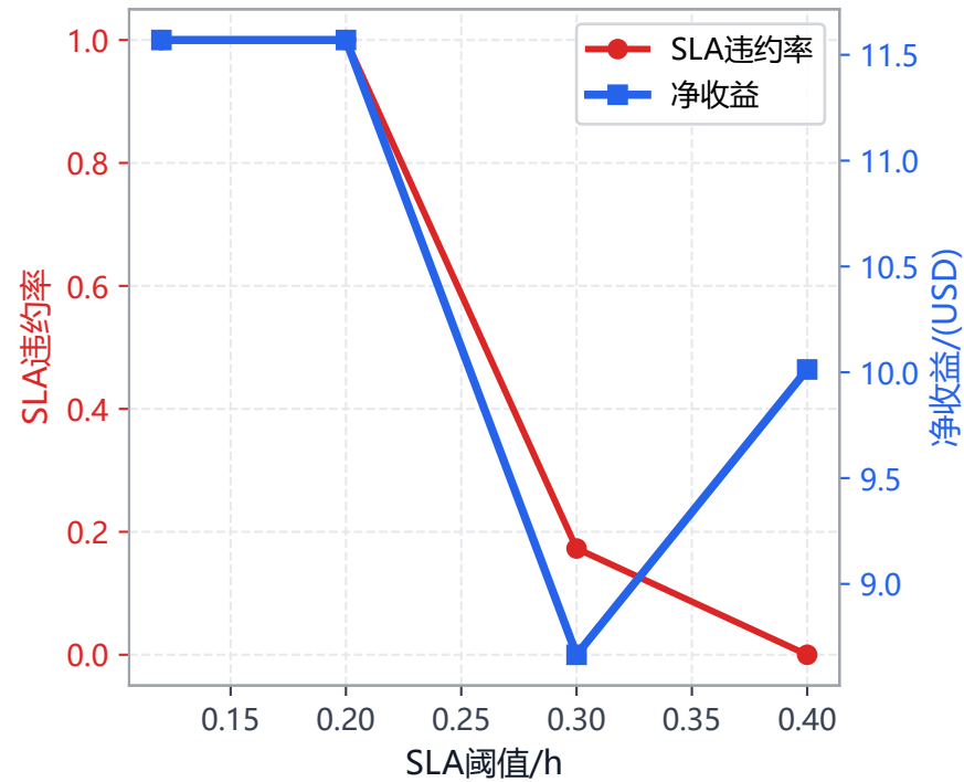
SLA阈值敏感性
