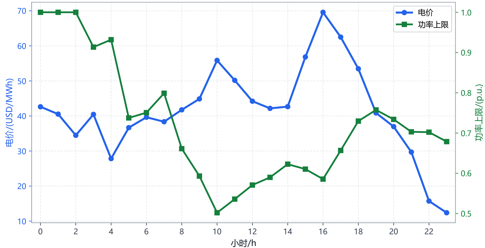
电价与功率上限关系
