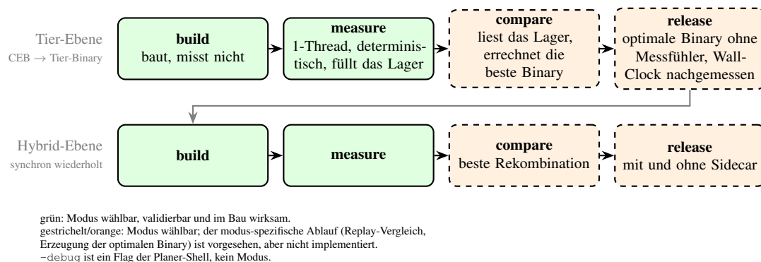
Abbildung 3.5: Die Ablauf-Kette der vier Arbeitsmodi build → measure → compare → release als registrierte Unter-Achse des Mess-Realms, kumulativ in dieser Reihenfolge und auf der Hybrid-Ebene synchron wiederholt; compare liest das Messwertlager und errechnet die beste Binary bzw. Rekombination, release erzeugt die voll optimierte Binary ohne Messfühler und misst ihre Wall-Clock nach. Ein Debug-Zustand existiert nicht. Die Zuordnung zu den Betriebs-Zielbildern Mess-, Auswertungs-, Arbeits- und Hybrid-Modus gibt Abschnitt 3.6.2.
