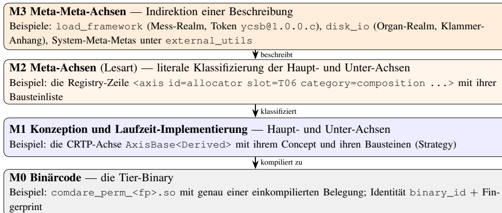
Abbildung 4.5: Die vier Abstraktionsebenen M0–M3 als Lesart der Achsen-Begriffe, in Anlehnung an die Meta-Ebenen-Architektur der MOF: Meta-Meta-Achsen (M3) beschreiben, wie andere Achsen beschrieben werden; die Registry-Zeile (M2) klassifiziert Haupt- und Unter-Achsen; die CRTP-Achse (M1) ist ihre Konzeption und Laufzeit-Implementierung; die Tier-Binary (M0) ist der Binärcode genau einer Belegung.
