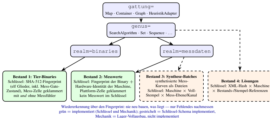
Abbildung 3.9: Das Lager: der Lager-Baum ist nach Gattung, Genus und Realm gegliedert; darunter liegen vier Bestände unter Stempel-Schlüsseln — Bestand 1 die Tier-Binaries (SHA-512-Fingerprint; die Binary mit und die ohne Messfühler sind zwei Einträge, weil der Mess-Gate-Zustand ein Fingerprint-Glied ist), Bestand 2 die Messwerte (Fingerprint der Binary plus Hardware-Identität der Maschine), Bestand 3 die Synthese-Batches mit den synthetisierten Mess-Kurven als Dateien und Bestand 4 die Lösungen je Anwender-XML. Der Apparat erkennt Vorhandenes über den Fingerprint wieder und misst nur Fehlendes nach.
