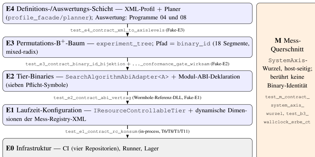
Abbildung 4.4: Die Ebenen E4–E0 des Schichtenmodells (Abschnitt 3.3.4) an ihrem Ort im Code, mit dem Contract-Test je Grenze (Fake der Nachbar-Ebene) und dem Mess-Querschnitt M, der alle Ebenen host-seitig quert, ohne die Binary-Identität zu berühren.
