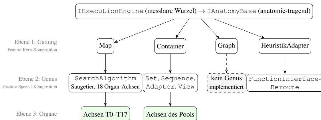
Abbildung 3.2: Das Drei-Ebenen-Modell: Gattung (Ebene 1, Außen-Interface, Feature-Kern-Komposition) → Genus (Ebene 2, fester Achsen-Satz, Feature-Spezial-Komposition) → Organe/Achsen (Ebene 3). Vier Gattungen: Map besitzt als einziges Genus SearchAlgorithm das „Säugetier“ mit den achtzehn Organ-Achsen; Container die Genera Set/Sequence/Adapter/View, die aus demselben Achsen-Pool gebildet werden; Graph ist als Interface angelegt, ein Genus ist nicht implementiert; HeuristikAdapter besitzt das Reroute-Genus FunctionInterfaceReroute des Hybrid-Tiers.
