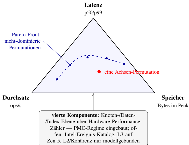
Abbildung 3.8: Das Mess-Trade-off-Dreieck: jede Achsen-Permutation spannt sich gegen die drei gegenläufigen Mess-Komponenten Latenz, Durchsatz und Speicherverbrauch auf und ist ein Punkt in seinem Inneren (vgl. den Entwurfsraum in Abbildung 3.1, wo dieselbe Permutation ein Punkt ist); die Pareto-Front der nicht-dominierten Permutationen ist die Brücke von den drei Größen zur „besten Binary“. Die für cache-bewusste Suchstrukturen zentrale vierte Komponente — das Verhalten auf Knoten-, Daten- und Index-Ebene über Hardware-Performance-Zähler — ist im Mess-Pfad verbindlich eingebaut; offen sind der Intel-Ereignis-Katalog, der Last-Level-Zähler auf Zen 5 und die nur modellgebundene L2-/Kohärenz-Belegung.
