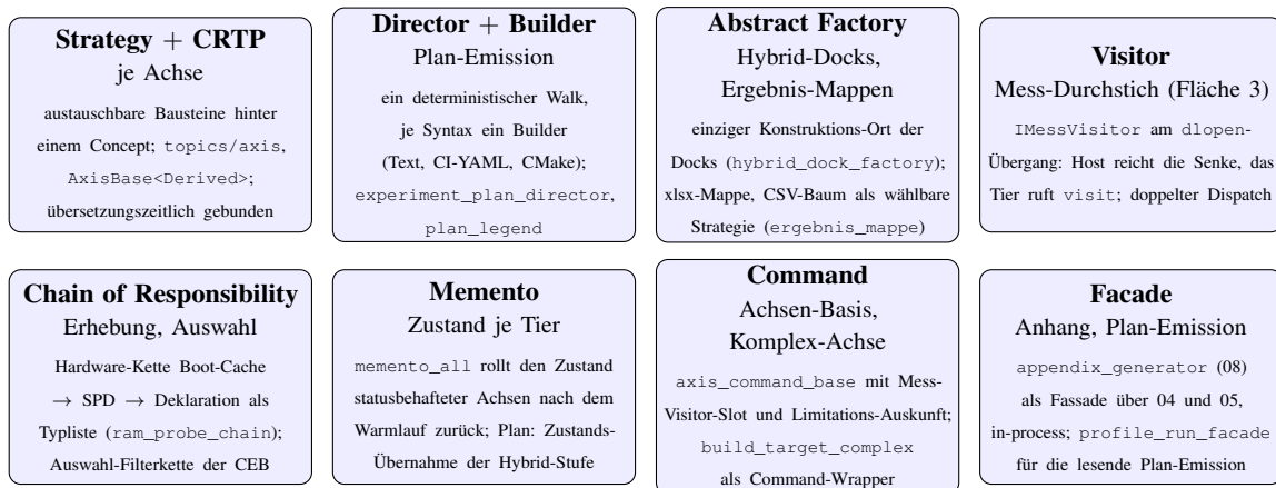
Abbildung 4.7: Das Register der Entwurfsmuster des Apparats (Benennung nach Gamma et al.): je Muster die Rolle und der Code-Ort. Alle acht sind übersetzungszeitlich ausgeführt — Bindung über Concepts, CRTP und Typlisten statt über virtuelle Aufrufe —, weil Tier-Binaries keine Laufzeit-Verzweigung zwischen Bausteinen enthalten dürfen.
