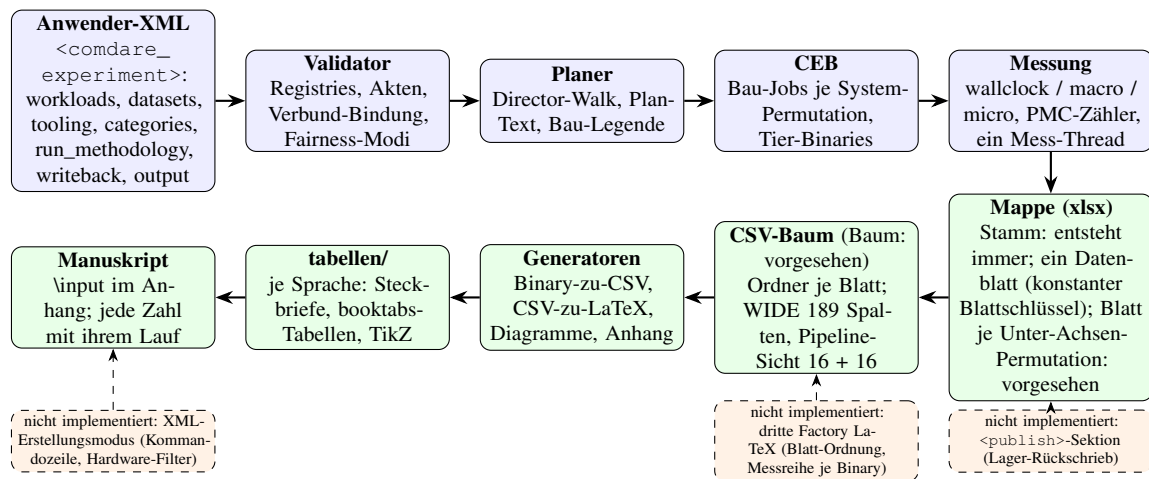
Abbildung 5.1: Die automatisierte Evaluations-Kette von der Anwender-XML bis zum Manuskript. Obere Reihe: Die XML deklariert Was, Wo und Wann; der Validator prüft sie gegen die Registries; der Planer emittiert den deterministischen Plan; die CEB baut je System-Permutation die Tier-Binaries; die Messung erhebt die drei Mess-Ebenen und die Zähler mit einem Mess-Thread. Untere Reihe: Die Mappe ist der Stamm (ein Datenblatt unter konstantem Blattschlüssel; die Auffächerung in ein Blatt je Unter-Achsen-Permutation ist vorgesehen, aber nicht implementiert), die CSV-Form ihr aus ihr erzeugter, geordneter Baum aus CSV-Dateien (ein Ordner je Blatt; kein einzelnes Kind-Dokument; implementiert ist eine flache Datei), die Generatoren rendern je Sprache in das tabellen-Verzeichnis, das Manuskript bindet die Dateien ein — jede Zahl führt ihren Lauf. Gestrichelt: nicht implementierte Teile (XML-Erstellungsmodus, <publish> -Sektion, dritte Factory).
