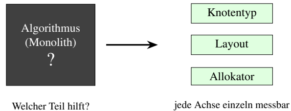
Abbildung 1.1: Das Trennbarkeits-Problem: als Monolith bleibt unklar, welche Entwurfsentscheidung wirkt; erst die Zerlegung in orthogonale Achsen macht jeden Beitrag isoliert messbar.
