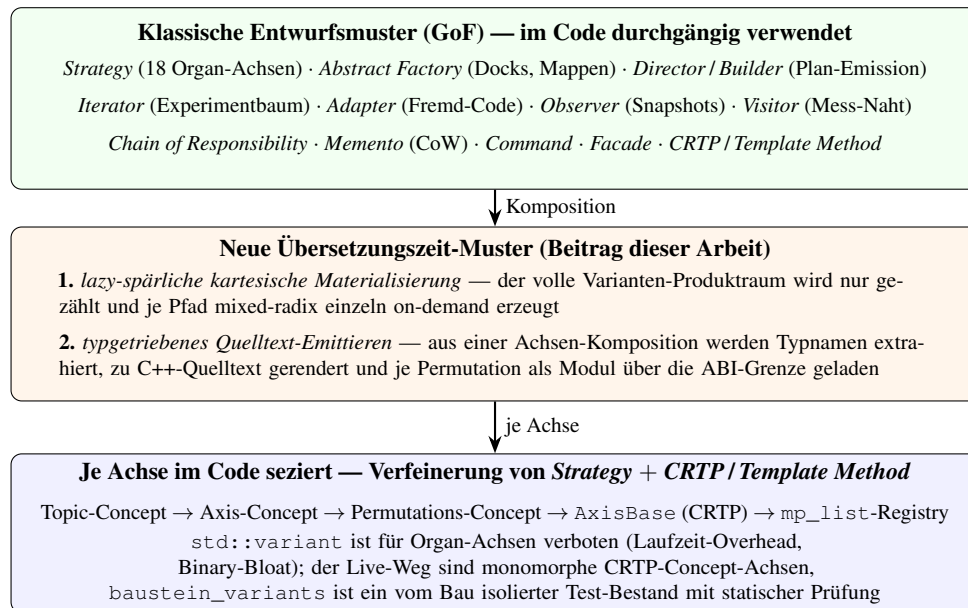
Abbildung 3.6: Entwurfsmuster als Bausteine der Architektur: oben die im Code durchgängig verwendeten klassischen GoF-Muster mit ihrer jeweiligen Rolle, in der Mitte die zwei in dieser Arbeit benannten neuen Übersetzungszeit-Muster, unten die code-seziert Drei-Stufen-Concept-Kette je Achse (Topic-Concept → Axis-Concept → CacheEngine-Permutations-Concept → CRTP-Basis → mp_list-Registry) als Verfeinerung von Strategy / CRTP ; ein literaler std::variant tritt in keiner Organ-Achse auf (Verbot), sondern nur in einem vom Bau isolierten Test-Bestand. Ihre Komposition bildet die design-pattern-getriebene, mess-orientierte Architektur (Kapitel 4).
