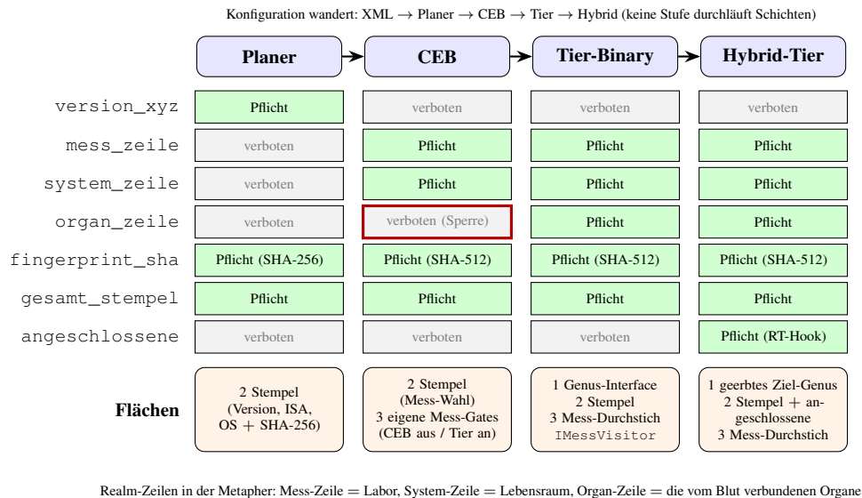
Abbildung 3.4: Träger-Stufen und Interface-Flächen: die dreiwertige Zulassungsmatrix der sieben Stempel-Interfaces über die vier Träger-Stufen Planer, CacheEngineBuilder (CEB), Tier-Binary und Hybrid-Tier-Binary (28 Zellen; grün = Pflicht, grau = verboten; die Zelle Organ-Zeile/CEB ist die statische Sperre „der CEB führt keine Organ-Achsen“) und darunter die Interface-Flächen je Stufe — Fläche 1 Genus-Interface (Laufzeit), Fläche 2 Stempel (Übersetzungszeit, ABI-stabil), Fläche 3 Mess-Durchstich. Die Konfiguration wandert von der XML über Planer und CEB bis zur Tier-Binary; keine Stufe durchläuft Schichten, jede enthält ihre Schicht einkompiliert.
