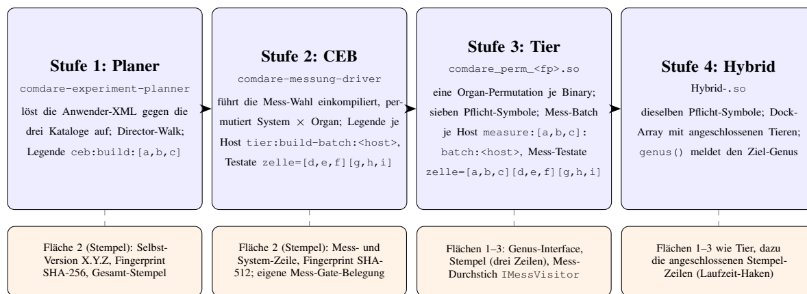
Abbildung 4.1: Die Träger-Stufenkette im Code: vier Träger in fester Reihenfolge (Stempel-Vertrag), je Stufe die Binary, ihre Legenden-Form in der emittierten Pipeline und die an ihr ausgeprägten Vertrags-Flächen. Stufe N + 1 hängt nur an Stufe N ; nur die Mess-Testate enthalten alle drei Achsen-Klammern. Die Flächen zergliedern die Verträge (Abschnitt 4.3.2); die Unterprojekte unter libs/traeger sind ein Gerüst, die Implementierung liegt als Monolith unter libs/cache_engine .
