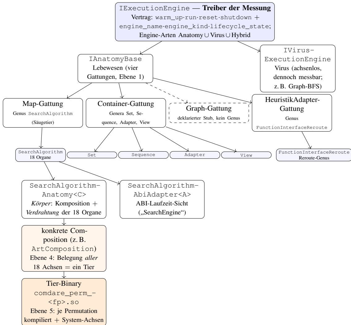
Abbildung 4.2: Die eine Architektur als einzige Hierarchie ohne Parallel-Bäume. An der Wurzel steht IExecutionEngine als Treiber der Messung — der universelle messbare Vertrag aus Mess-Lebenszyklus (warm_up/run/reset/shutdown) und Auskünften (engine_name/engine_kind/lifecycle_state) über alle drei Engine-Arten Anatomy, Virus und Hybrid; unter ihm verzweigen die anatomie-tragenden Gattungen (Ebene 1: Map, Container, Graph, HeuristikAdapter) mit ihren Genera (Ebene 2) und die achsenlosen Viren . SearchAlgorithm ist das fokale Lebewesen (Säugetier); seine Anatomie ist sein Körper — die feste Komposition und Verdrahtung der 18 Organe —, und „SearchEngine“ nur dessen ABI-Laufzeit-Sicht. Der Säugetier-Ast ist bis zum Individuum ausgezogen: eine konkrete Achsen-Composition (Ebene 4) wird je Permutation als eigenständige Tier-Binary kompiliert (Ebene 5). Container besitzt einen eigenen Organsatz mit den Genera Set, Sequence, Adapter und View, deren Aritäten die Genus-Bau-Zulassung führt; Graph ist deklariert und besitzt keinen Genus; die Gattung HeuristikAdapter führt das Reroute-Genus der Hybrid-Stufe.
