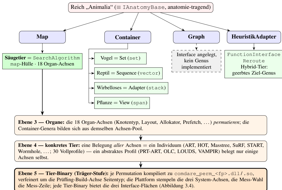
Abbildung 3.3: Die Gattungs-/Tier-Hierarchie über fünf Ebenen. Map, Container, Graph und HeuristikAdapter sind die vier Gattungen (Ebene 1, Außen-Interface). Jede Gattung beherbergt ihre eigenen Genera (Ebene 2, Alias Tier-Unterklassen): Map ausschließlich das „Säugetier“ (Genus SearchAlgorithm, volle Achtzehn-Achsen-Anatomie), Container jedes nicht -Säugetier-Genus (Vogel/Reptil/Wirbelloses/Pflanze = Set/Sequence/Adapter/View), Graph ein angelegtes Interface ohne implementiertes Genus, HeuristikAdapter das Reroute-Genus des Hybrid-Tiers. Der Säugetier-Ast ist bis zum Individuum ausgezogen: die achtzehn Achsen-Organen (Ebene 3) permutieren zu einer konkreten Achsen-Komposition = einem konkreten Tier (Ebene 4, z. B. ART, HOT, Masstree), das je Permutation als eigenständige Tier-Binary kompiliert wird (Ebene 5, die Träger-Stufe der Tier-Binary, zusätzlich verfeinert um die Prüfling-Build-Achse Seitentyp und plattform-gestempelt durch die drei System-Achsen, Abschnitt 3.4.1). Jede Tier-Binary ist damit ein eigenes Tier mit einem tatsächlichen Binary-Genus-Interface und drei Interface-Flächen ; die Hierarchie reicht von der Gattung bis zur einzelnen kompilierten Permutation. Vgl. das verdichtete Modell in Abbildung 3.2.
