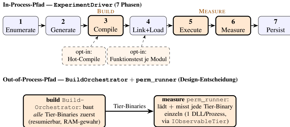
Abbildung 4.3: Die Mess-Pipeline in zwei Ausprägungen. Der In-Process-Pfad (oben) ist die Sieben-Phasen-Pipeline des ExperimentDriver je Messreihe (Enumerate → Generate → Compile → Link+Load → Execute → Measure → Persist; zwei opt-in-Phasen kompilieren fehlende Module im laufenden Experiment nach und fahren je Modul einen Funktionstest mit ABI-Versionsprüfung). Hervorgehoben sind die substantziellen Phasen: COMPILE (der Build der Tier-Binaries) und EXECUTE/MEASURE (die Messung ); Generate/Link+Load/Persist sind Verdrahtung. Der Out-of-Process-Pfad (unten) ist eine Design-Entscheidung zur Prozess-Isolation: Der BuildOrchestrator baut zuerst alle Tier-Binaries (resumierbar, RAM-gewahr), danach lädt und misst perm_runner jede Binary einzeln über die Beobachter-Schnittstelle IObservableTier — eine DLL je Prozess, weil die DLL kein main enthält und der Runner das Executable ist, das sie lädt; kein Zustand wird zwischen Permutationen geteilt, und eine Cluster-Task fährt genau einen Runner mit genau einer DLL.
