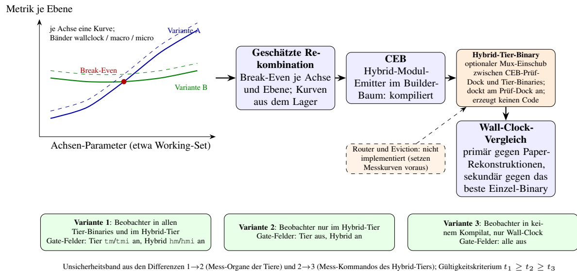
Abbildung 5.3: Das Messkurven-Typsystem im heuristischen Gegenbeweis. Links: je Achse eine Kurve der Metrik über dem Achsen-Parameter, getrennt nach Mess-Ebene (wallclock, macro, micro); der Schnittpunkt zweier Varianten ist der Break-Even-Punkt, aus dem die Rekombination geschätzt wird. Mitte und rechts: Die CEB kompiliert die geschätzte Rekombination über den Hybrid-Modul-Emitter; die Hybrid-Tier-Binary ist die optional zwischen CEB-Prüf-Dock und Tier-Binary eingeschobene Mux-Stufe, dockt am Prüf-Dock an, führt Dock-Slots für Tier-Binaries und erzeugt selbst keinen Code; verglichen wird an der Wall-Clock, primär gegen die Paper-Rekonstruktionen, sekundär gegen das beste Einzel-Binary. Unten: die drei Bau-Varianten des Messfehler-Prüfplans, auseinandergehalten über die Gate-Felder des Fingerprints. Gestrichelt: Router und Eviction (nicht implementiert).
