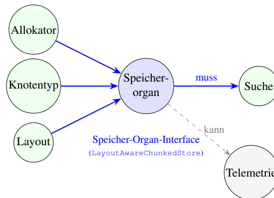
Abbildung 3.5: Achse = Organ, Anatomie = Verdrahtung: das Speicher-Organ (Komposition aus Knotentyp, Layout und Allokator) exportiert ein generalisiertes Speicher-Organ-Interface (im Code LayoutAwareChunkedStore ), über das die Suche läuft (durchgezogen, verpflichtend ); weitere Organe wie die Telemetrie können es über optionale Beobachter-Hooks nutzen (gestrichelt, optional ), müssen aber nicht.
