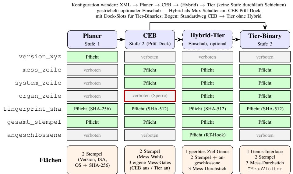
Abbildung 3.9: Träger-Stufen und Interface-Flächen: die dreiwertige Zulassungsmatrix der sieben Stempel-Interfaces über die vier Träger-Stufen Planer, CacheEngineBuilder (CEB), Hybrid-Tier-Binary (optionaler Einschub) und Tier-Binary (28 Zellen; grün = Pflicht, grau = verboten; die Zelle Organ-Zeile/CEB ist die statische Sperre „der CEB führt keine Organ-Achsen“) und darunter die Interface-Flächen je Stufe — Fläche 1 Genus-Interface (Laufzeit), Fläche 2 Stempel (Übersetzungszeit, ABI-stabil), Fläche 3 Mess-Durchstich. Die Konfiguration wandert von der XML über Planer und CEB bis zur Tier-Binary; die Hybrid-Tier-Binary ist eine optional zwischen CEB-Prüf-Dock und Tier-Binary eingeschobene Stufe (gestrichelt: Mux-Schalter am Prüf-Dock mit Dock-Slots für Tier-Binaries; die Spaltenordnung der Matrix folgt der Verarbeitungs-Topologie mit dem Hybrid an seiner Einschub-Position, der Bogen ist der Standardweg ohne Hybrid); keine Stufe durchläuft Schichten, jede enthält ihre Schicht einkompiliert.
