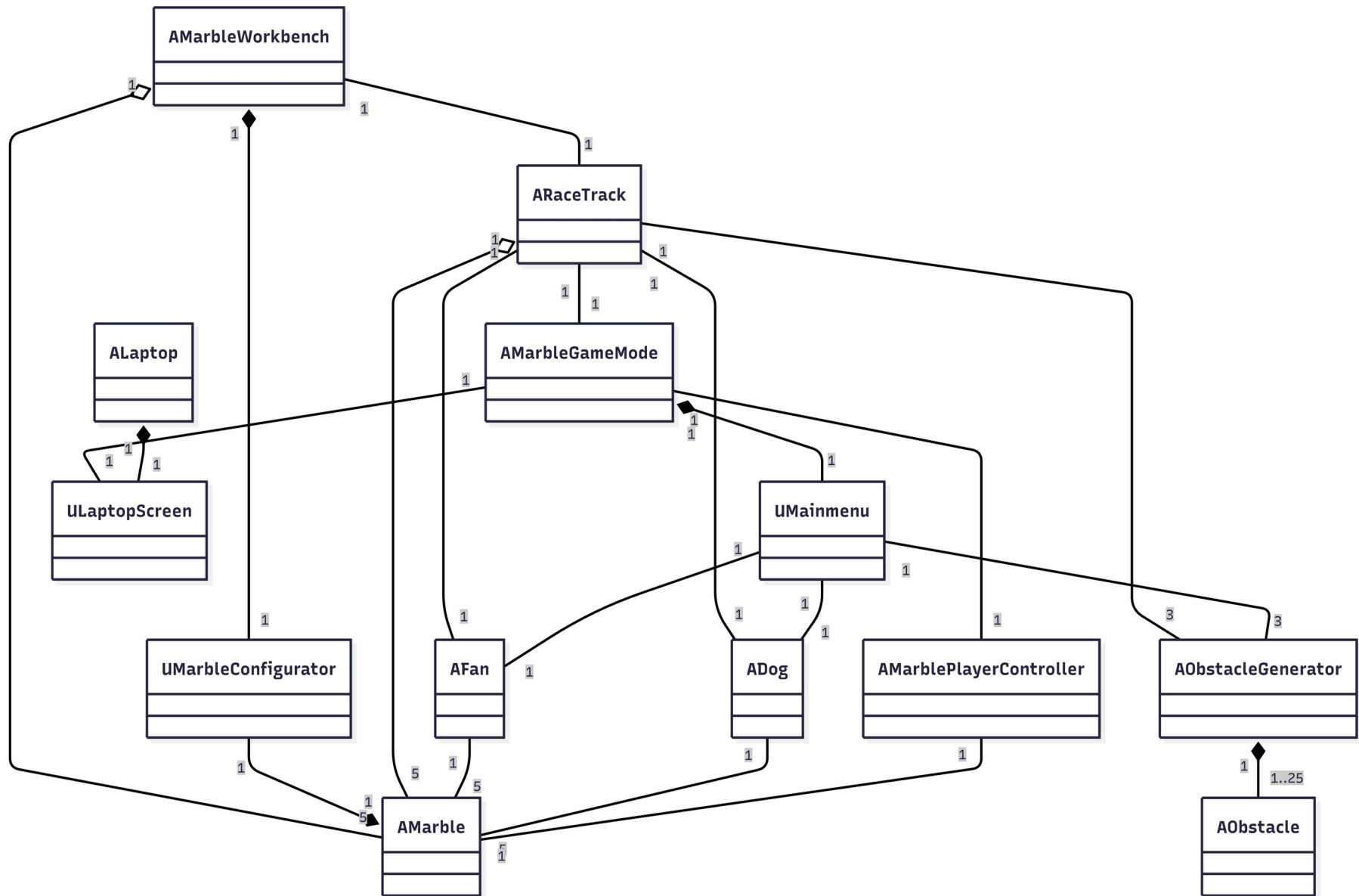
Schaubild 2: Klassendiagramm (nur die Beziehungen)
