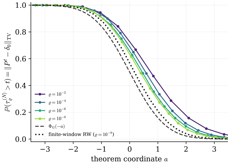
Finite-precision cutoff, N = 20 , A = 0.7
