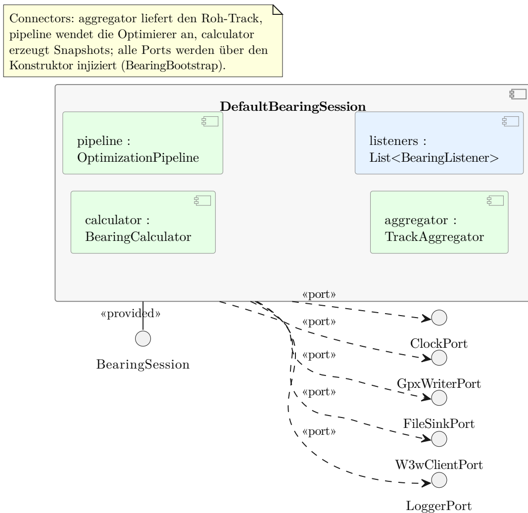
Abbildung 25: Kompositionsstrukturdiagramm: Innenleben von DefaultBearingSession .
