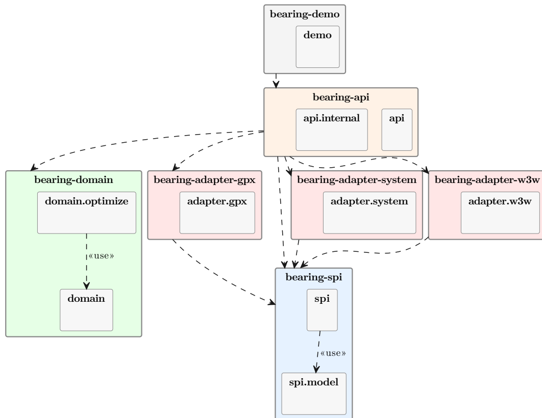
Abbildung 23: Paketdiagramm: Maven-Module und Java-Pakete mit ihren Abhängigkeiten.
