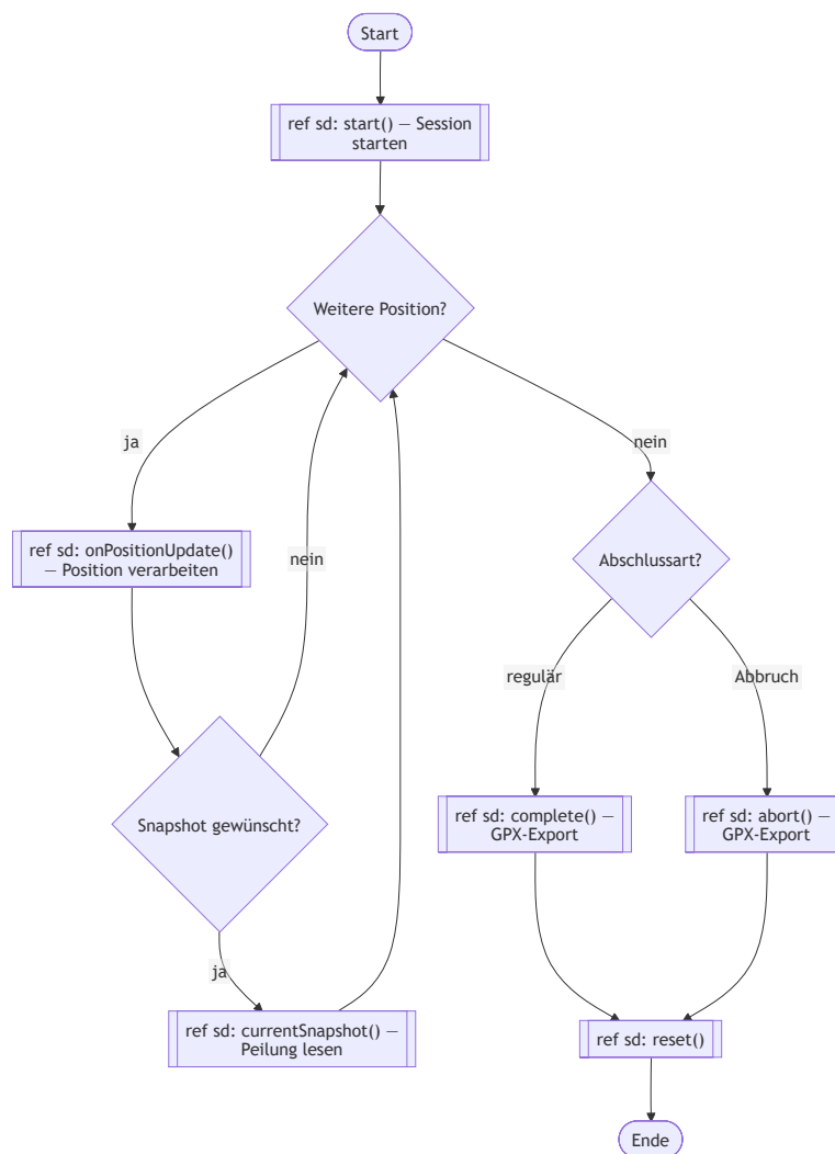
Abbildung 30: Interaktionsübersichtsdiagramm: Ablauf als Folge von Interaktionsverweisen.
