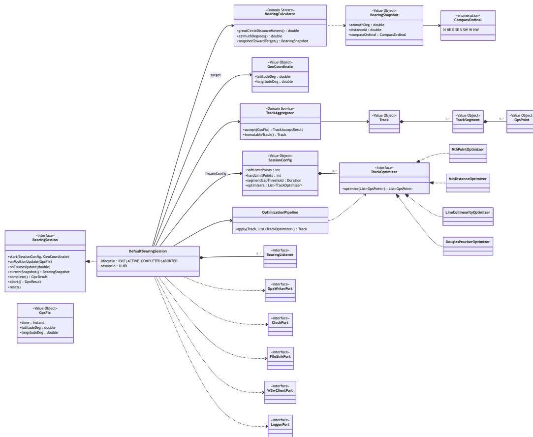
Abbildung 19: Klassendiagramm (OOD): Fassade, Value Objects, Domain Services, Strategy, Observer und Ports.
