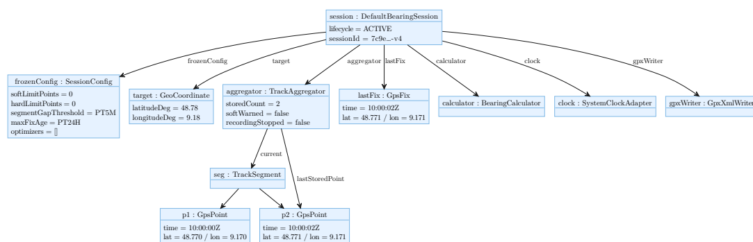
Abbildung 20: Objektdiagramm: Momentaufnahme einer aktiven Session (ACTIVE, zwei gespeicherte Punkte).
