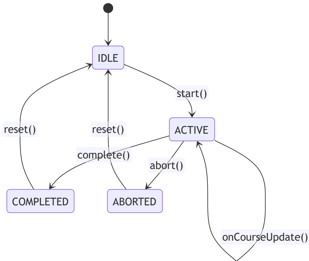
Abbildung 21: Zustandsdiagramm des Session-Lebenszyklus.
