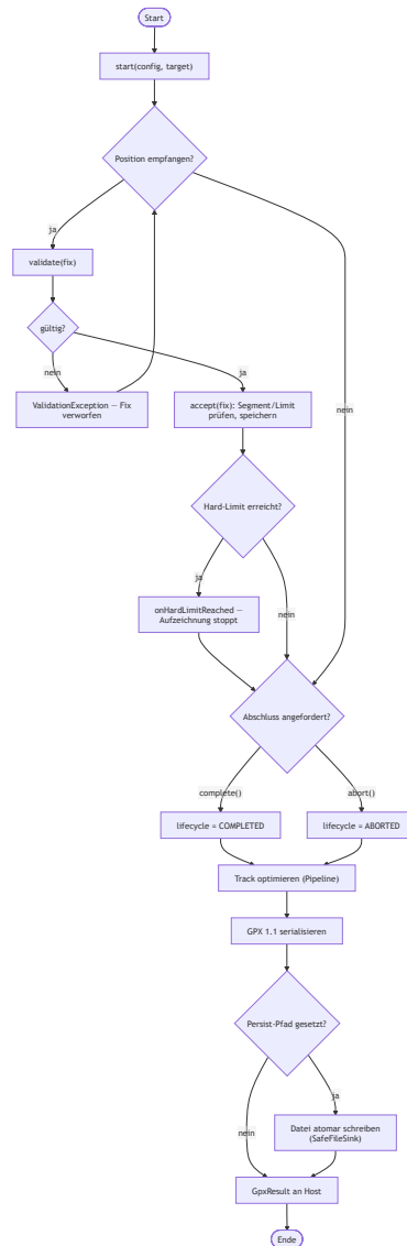
Abbildung 29: Aktivitätsdiagramm: vollständiger Verlauf einer Peilungssession.
