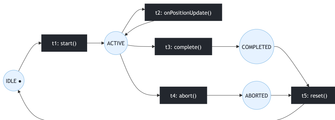
Abbildung 32: Petri-Netz des Session-Lebenszyklus (Stellen, Transitionen, eine Marke).
