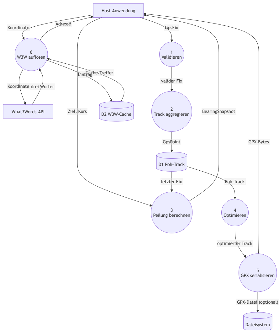
Abbildung 31: Datenflussdiagramm (DFD Stufe 1): Teilprozesse und Datenspeicher.
