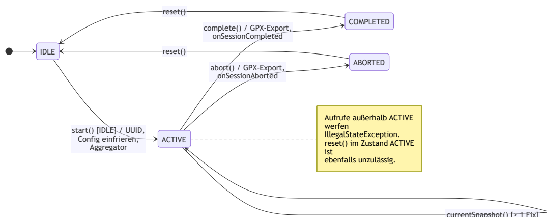
Abbildung 22: Zustandsdiagramm (detailliert) des Session-Lebenszyklus mit Guards und Effekten.
