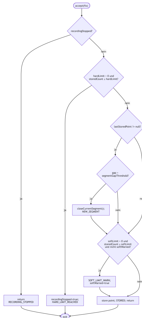
Abbildung 16: Kontrollflussgraph von TrackAggregator.accept
