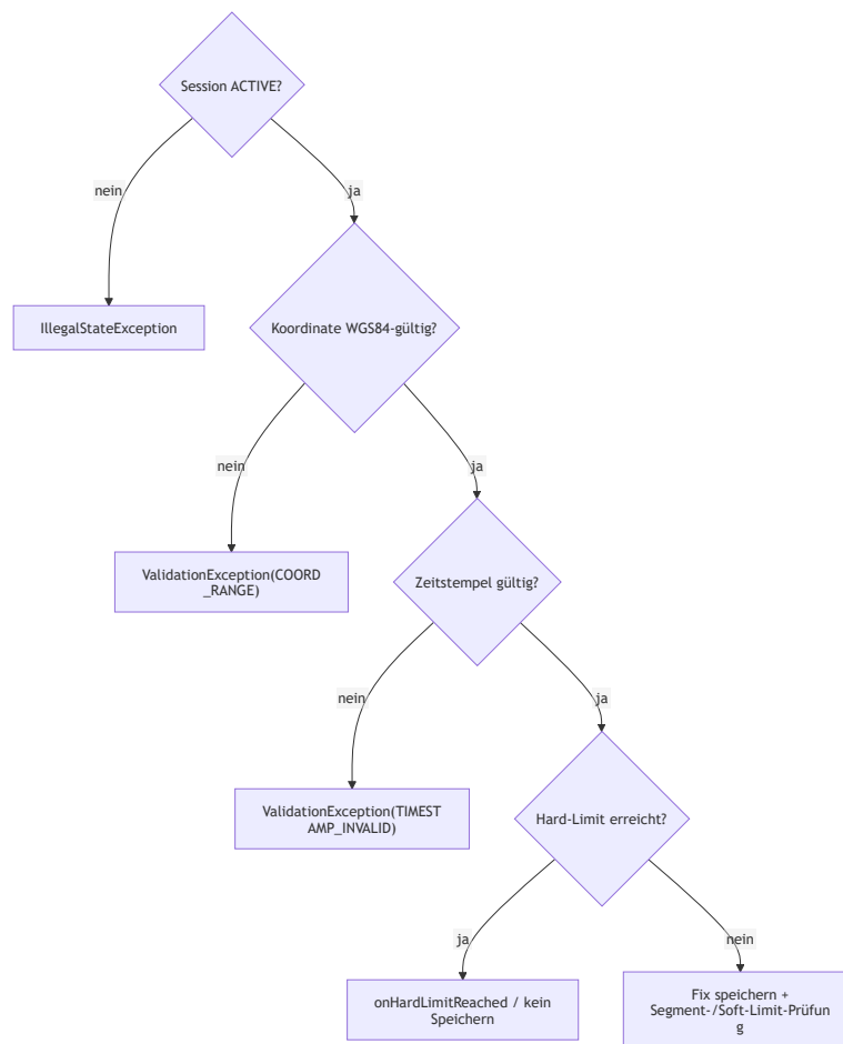
Abbildung 18: Entscheidungsbaum der Fix-Verarbeitung (Baumform der Entscheidungstabelle).
