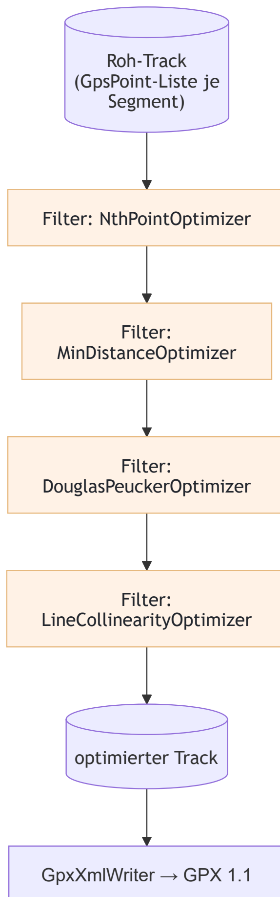
Abbildung 28: Architekturmuster Pipes-and-Filter: die Optimierer-Pipeline. Moritz Pfitzenmaier, Marius Müllmaier, Daniel Bensch
