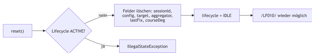
Abbildung 11: Aktivitätsdiagramm /LF090/
