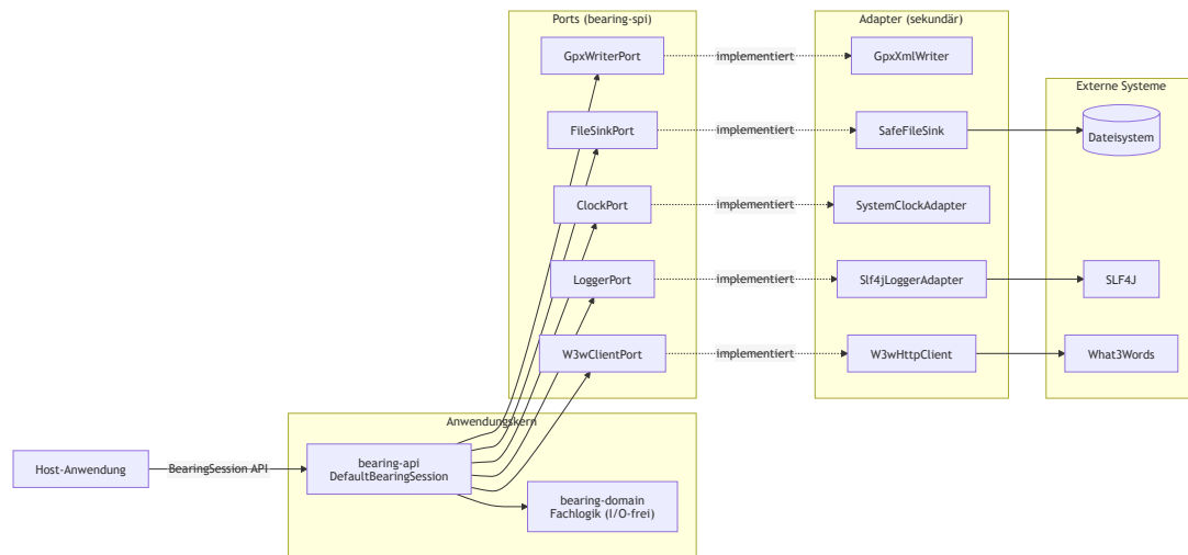
Abbildung 27: Architekturmuster Ports-and-Adapters (hexagonal).
