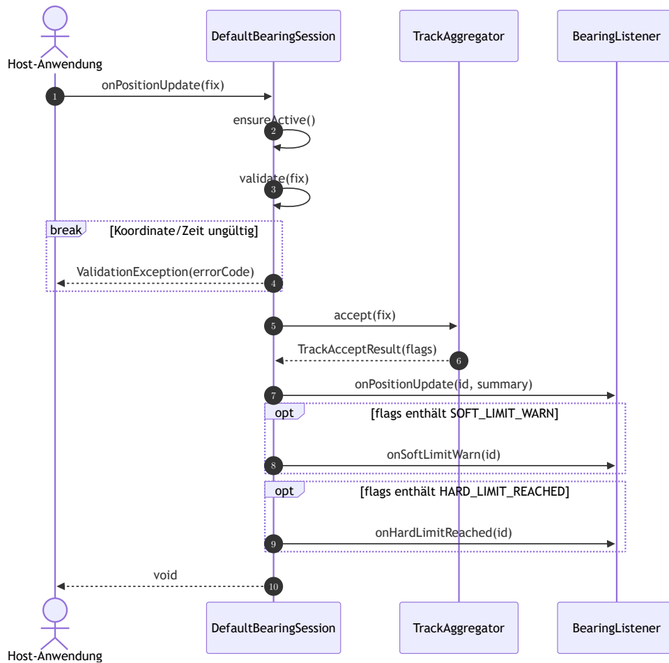
Abbildung 14: Sequenzdiagramm onPositionUpdate() : Validierung, Aggregation und Listener-Ereignisse (/LF030/).
