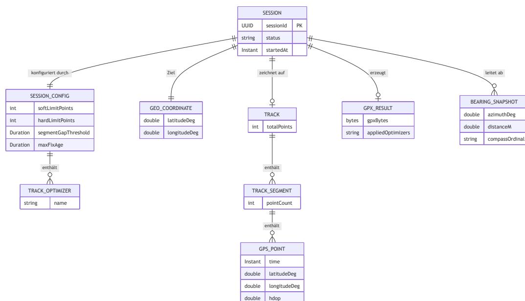
Abbildung 15: ER-Modell der Produktdaten (/LD010/ ... /LD060/) mit Entitäten und Kardinalitäten.
