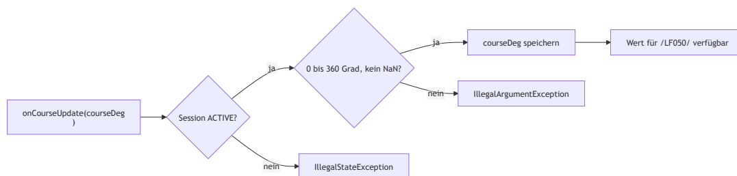
Abbildung 6: Aktivitätsdiagramm /LF040/
