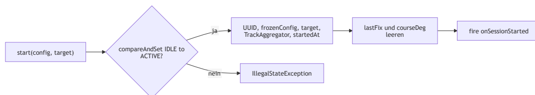
Abbildung 3: Aktivitätsdiagramm /LF010/
