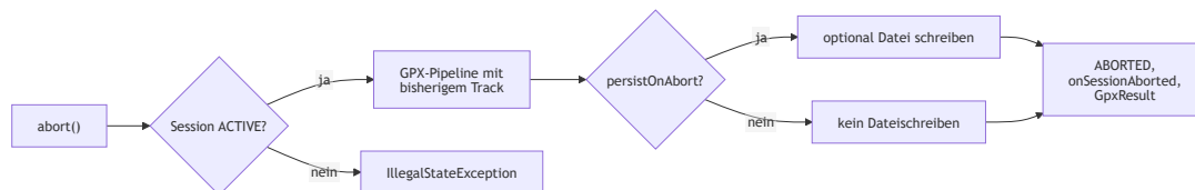
Abbildung 9: Aktivitätsdiagramm /LF070/
