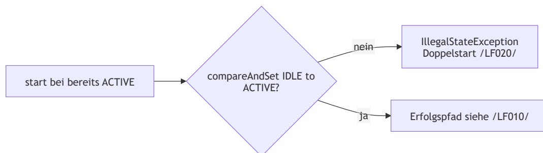
Abbildung 4: Aktivitätsdiagramm /LF020/
