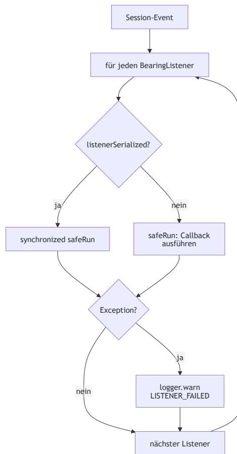
Abbildung 10: Aktivitätsdiagramm /LF080/
