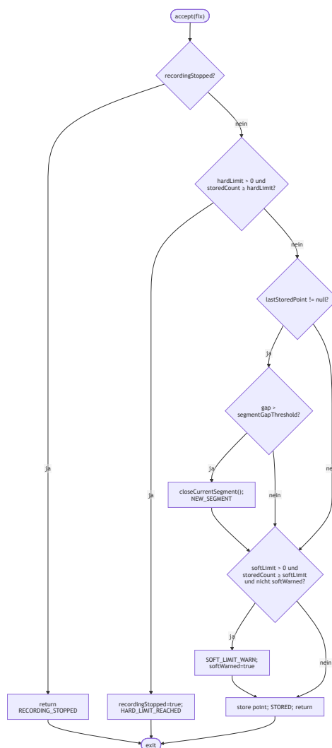
Abbildung 16: Kontrollflussgraph von TrackAggregator.accept (Whitebox-Sicht, v(G) = 6 ).
