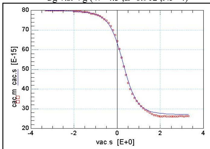
Cg v.s. Vg (W=4.5 ,L=0.912 ,NF=4)
