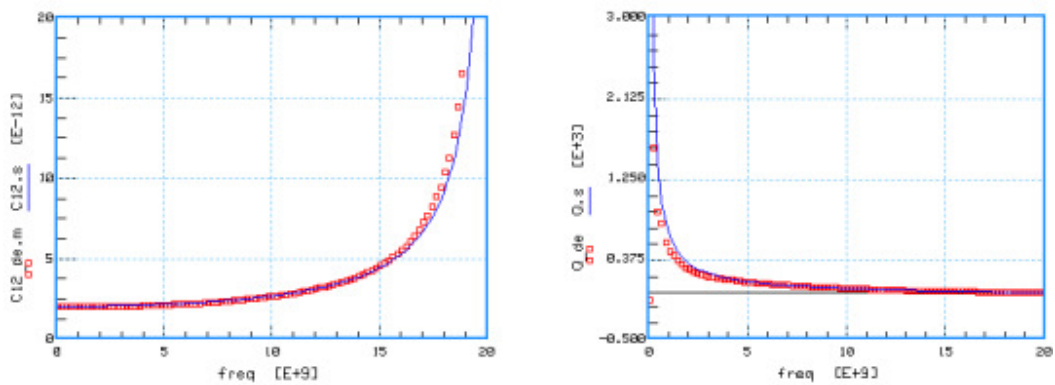
MMC6 : 50um x 50um
