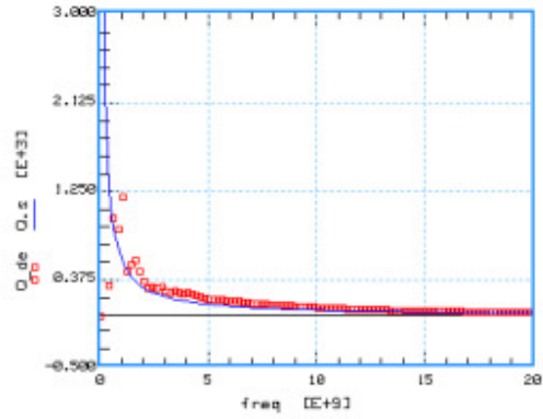
MMC4 : 10um x 10um
