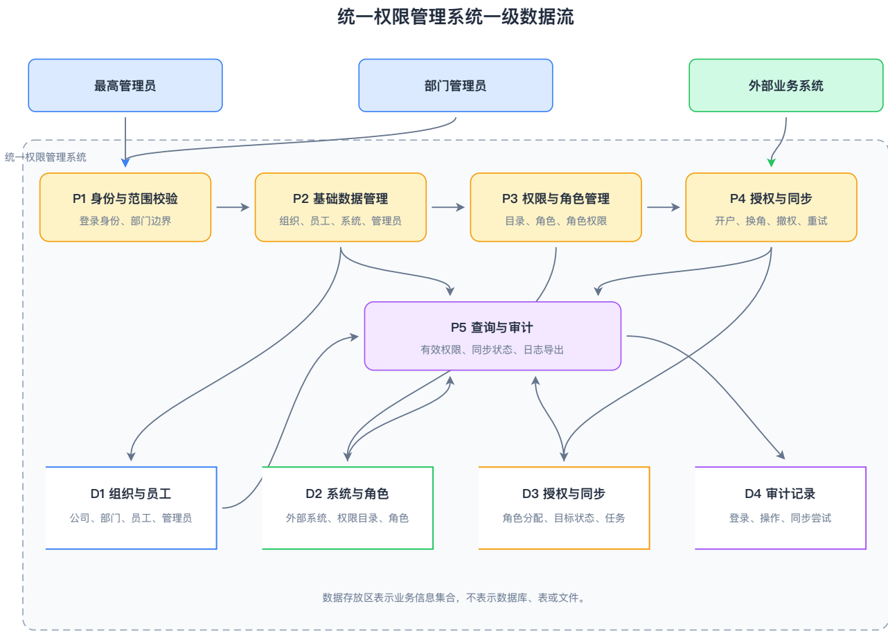
图 3-3 一级数据流图
