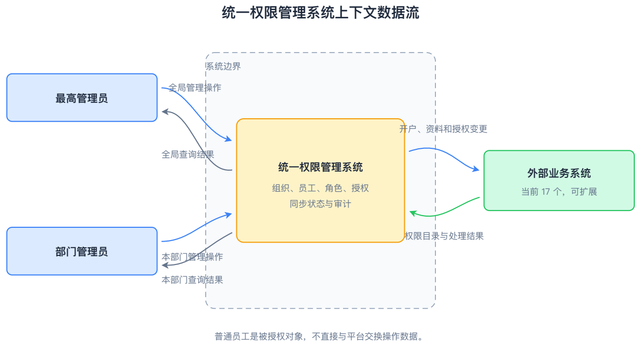
图 3-2 上下文数据流图
