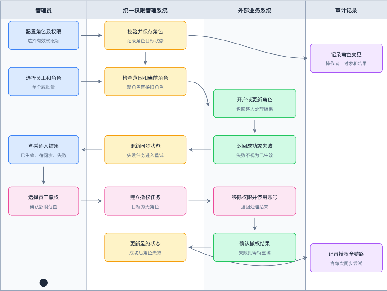
角色配置、开户授权和撤权流程
