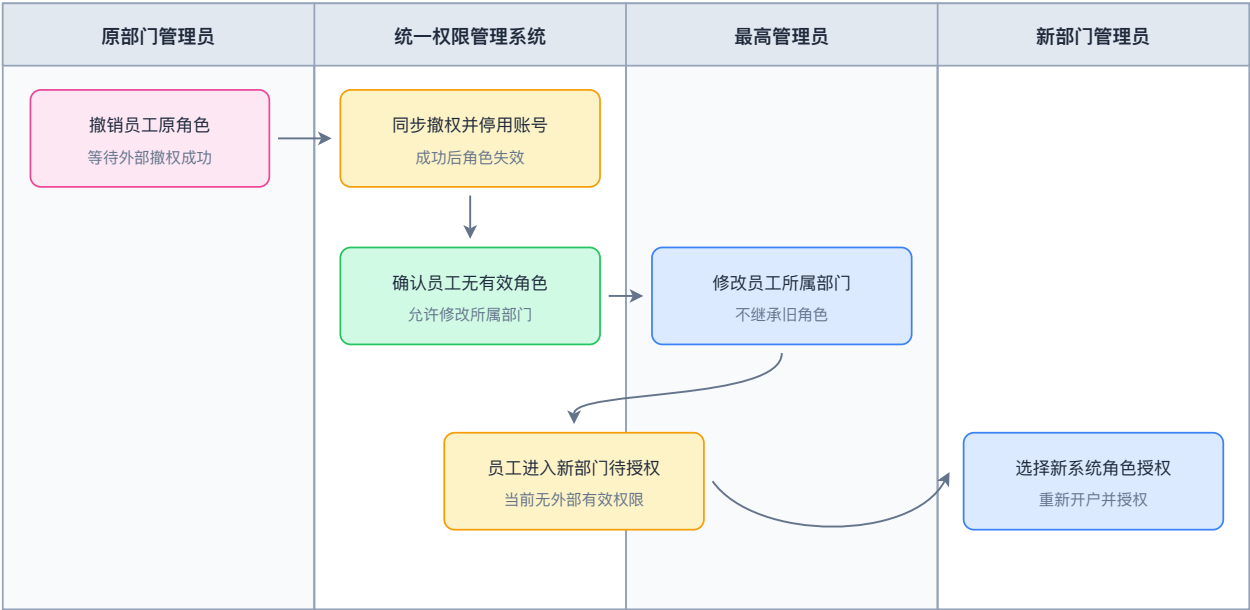
员工跨部门手工调动流程
