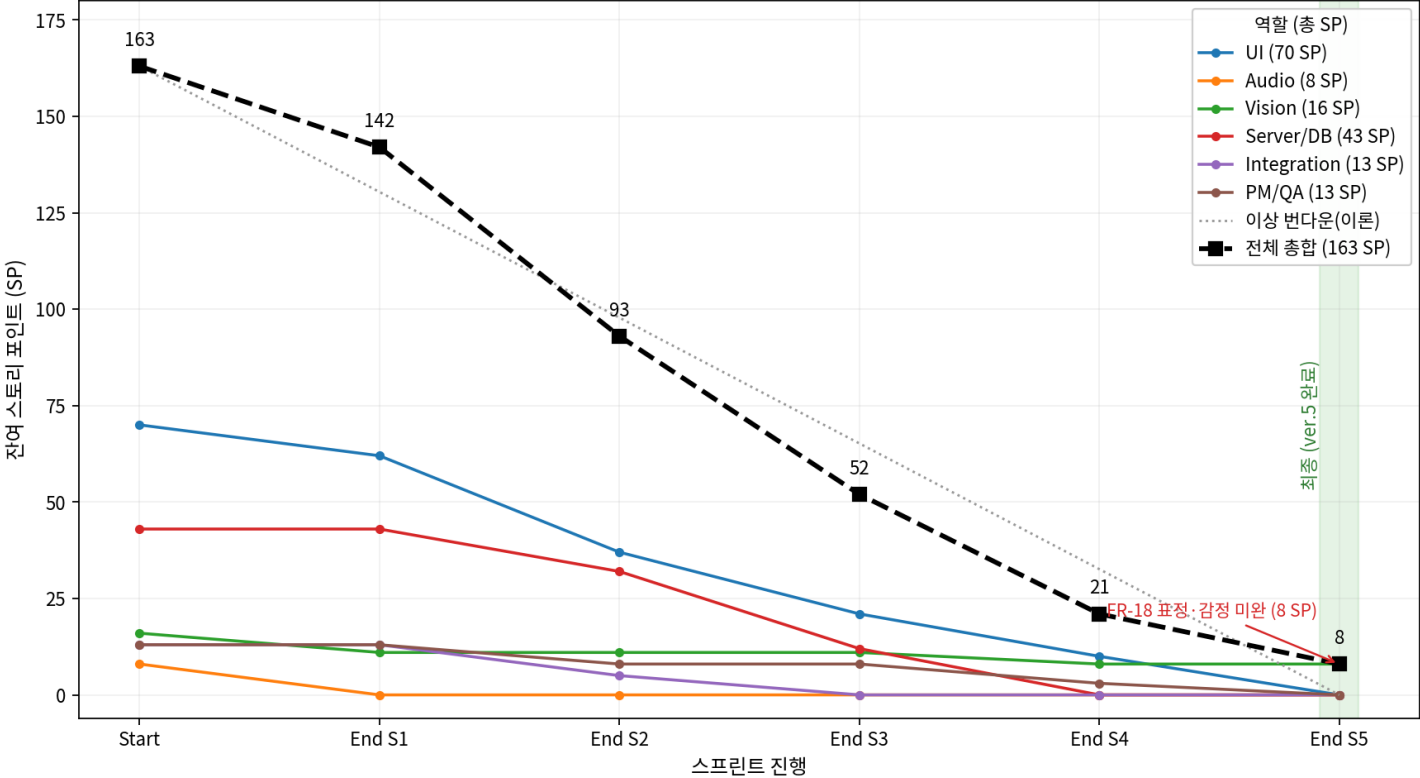
SpeechCoach AI — 6개 역할별 스프린트 번다운 차트 (Sprint 1~5)
