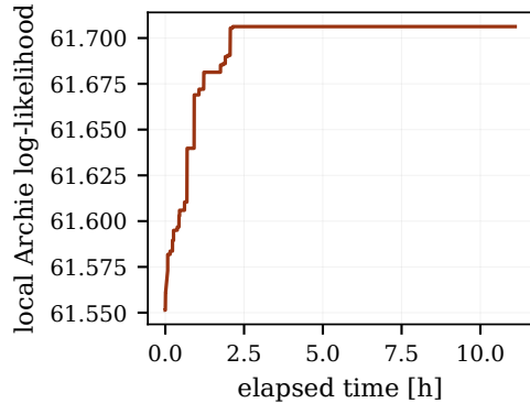
Best-so-far fit
