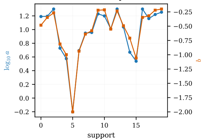
Best-fit local Archie parameters
