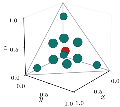
q11 (11 pts)
