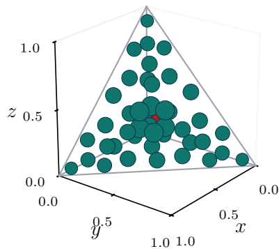
q45 (45 pts)
