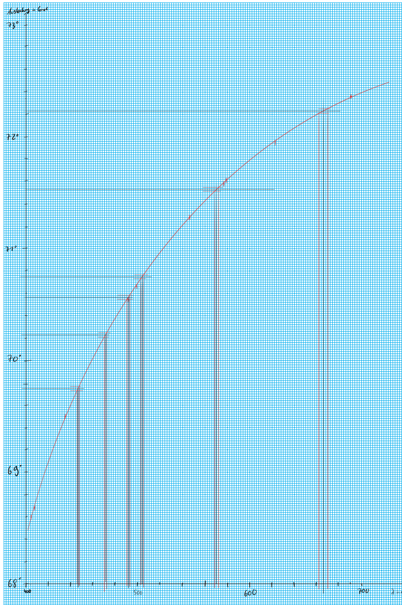
Abbildung 4: Bestimmung der Wellenlängen der He-Spektrallinien
