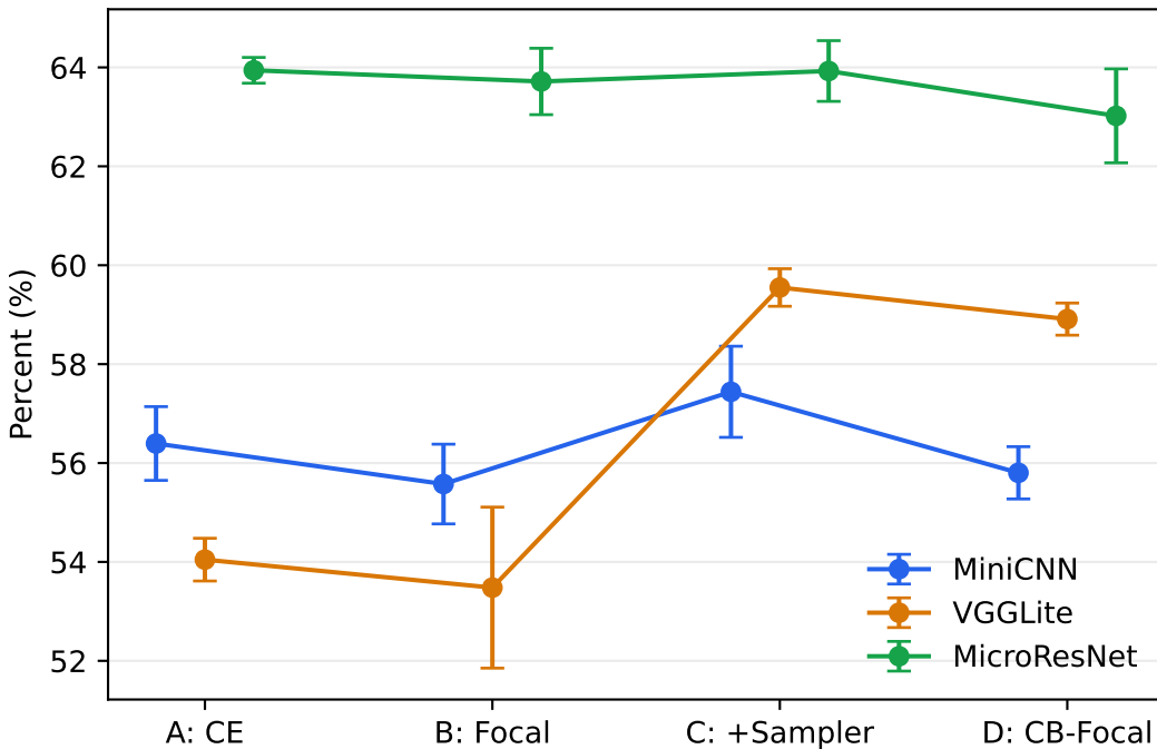
PublicTest macro-F1
