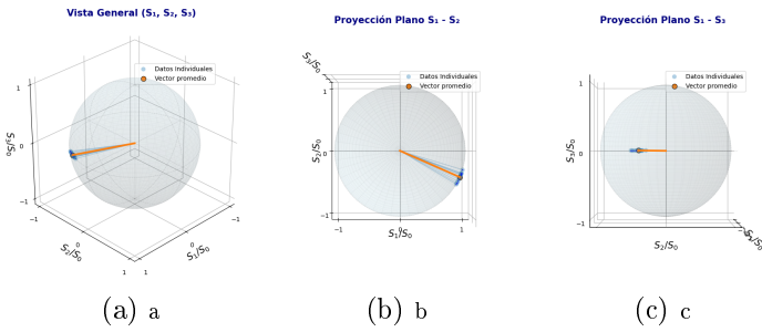
Figura 2: Se disponen diferentes visualizaciones de los vectores de Poincaré obtenidos para la polarización lineal correspondida a una inclinación de 0^\circ : (a) Vista general de los vectores, (b) Vista en el plano de los versores S_1 y S_2 , y (c) Vista en el plano de los versores S_3 y S_2
