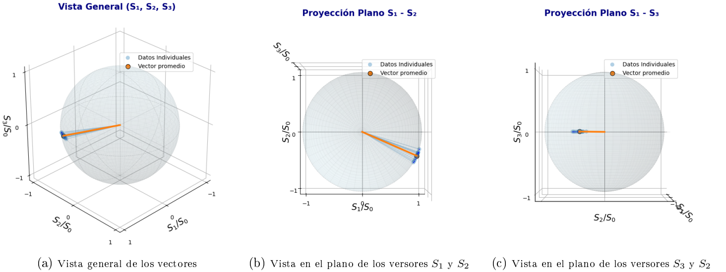
Figura 3: Se disponen diferentes visualizaciones de los vectores de Poincaré obtenidos para la polarización lineal correspondida a una inclinación de 0^\circ . Las figuras (a), (b) y (c) muestran distintas perspectivas de las mismas mediciones para facilitar la visualización.
