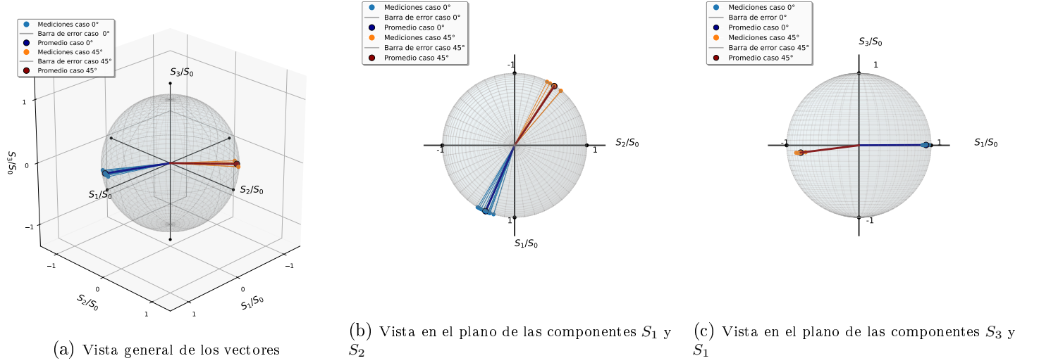
Figura 3: Se disponen diferentes visualizaciones de los vectores de Poincaré obtenidos para la polarización lineal correspondida a una inclinación de 0^\circ y 45^\circ de la lámina de media onda. Las figuras (a), (b) y (c) muestran distintas perspectivas de las mismas mediciones para facilitar la visualización.
