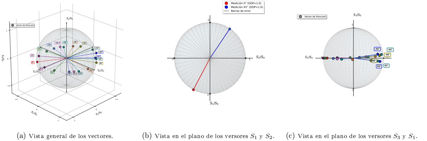
Figura 6: Se disponen diferentes visualizaciones de los vectores de Poincaré obtenidos para la polarización lineal correspondida distintas polarizaciones. Las referencias de ángulos corresponden a la rotación de la lámina de media onda. Las Figuras (a), (b), y (c) representan distintas perspectivas de la misma medición para facilitar la visualización.
