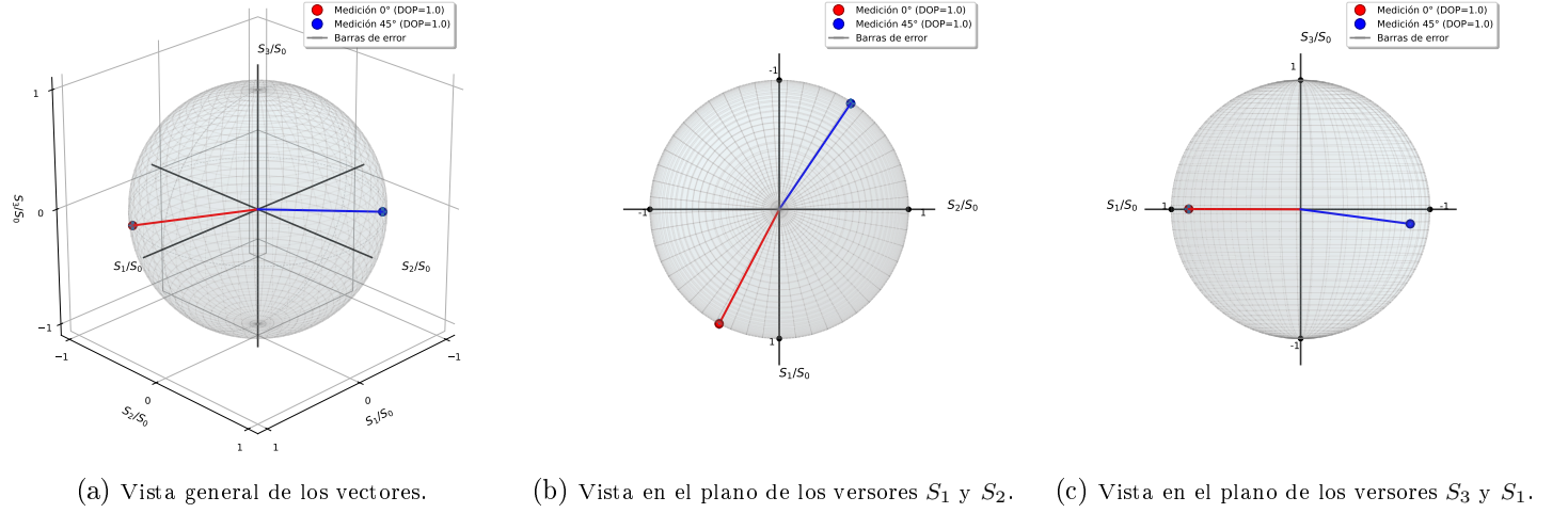
Figura 5: Se disponen diferentes visualizaciones de los vectores de Poincaré obtenidos para la polarización lineal correspondida a una inclinación de 0^\circ y 45^\circ . Las Figuras (a), (b), y (c) representan distintas perspectivas de la misma medición para facilitar la visualización.
