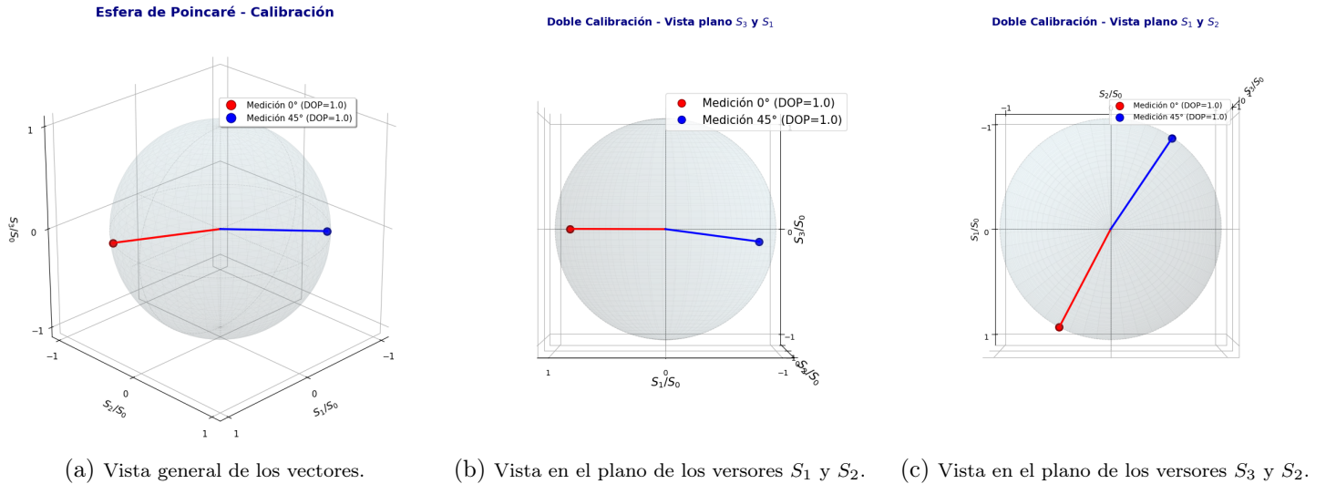
Figura 4: Se disponen diferentes visualizaciones de los vectores de Poincaré obtenidos para la polarización lineal correspondida a una inclinación de 0^\circ y 45^\circ . Las Figuras (a), (b), y (c) representan distintas perspectivas de la misma medición para facilitar la visualización.
