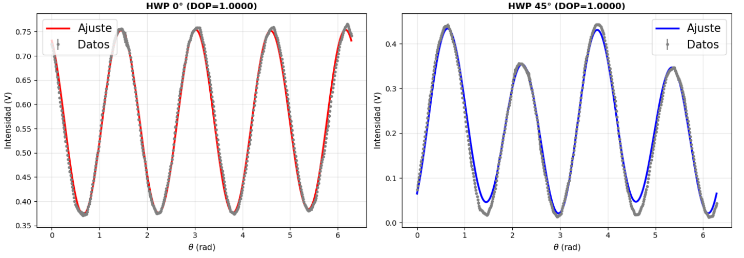
Figura 3: Se observa el ajuste realizado para las dos curvas, correspondientes a una rotación de la lámina de media onda de 0^\circ y 45^\circ respectivamente. Para ambos casos, el valor del DOP obtenido para cada vector de Stokes del par toma un valor de 1.
