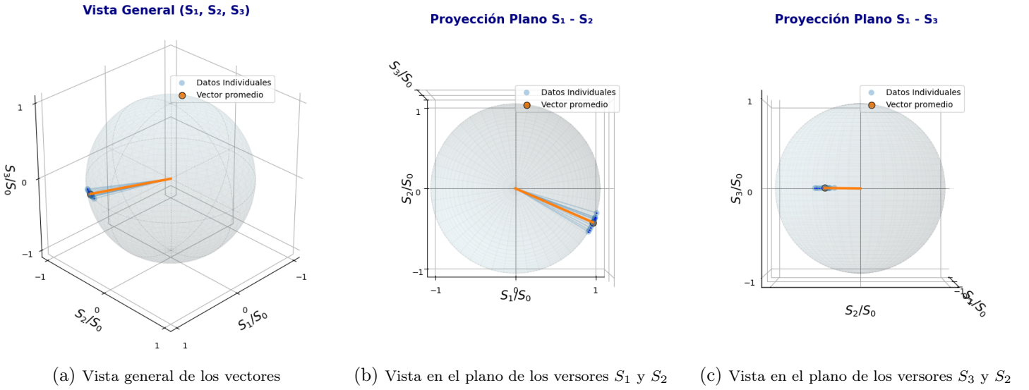
Figura 2: Se disponen diferentes visualizaciones de los vectores de Poincaré obtenidos para la polarización lineal correspondida a una inclinación de 0^\circ . Las figuras (a), (b) y (c) muestran distintas perspectivas de las mismas mediciones para facilitar la visualización.
