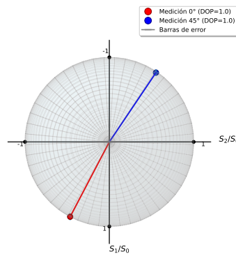
(b) Vista en el plano de los versores S_1 y S_2 .
