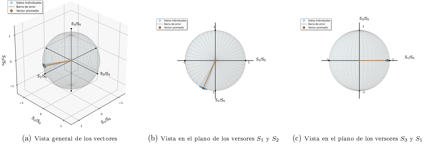
Figura 3: Se disponen diferentes visualizaciones de los vectores de Poincaré obtenidos para la polarización lineal correspondida a una inclinación de 0^\circ . Las figuras (a), (b) y (c) muestran distintas perspectivas de las mismas mediciones para facilitar la visualización.
