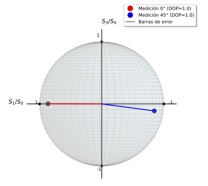
(c) Vista en el plano de los versores S_3 y S_1 .
