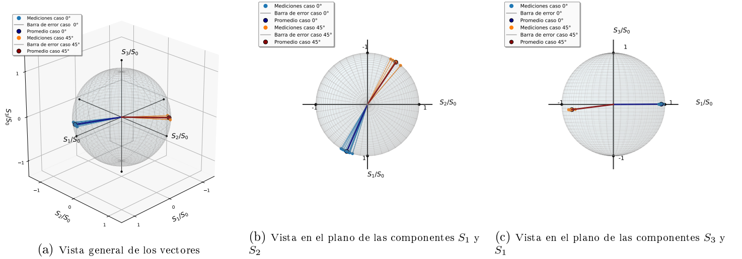
Figura 3: Se disponen diferentes visualizaciones de los vectores de Poincaré obtenidos para la polarización lineal correspondida a una inclinación de 0° y 45° de la lámina de media onda. Las figuras (a), (b) y (c) muestran distintas perspectivas de las mismas mediciones para facilitar la visualización.
