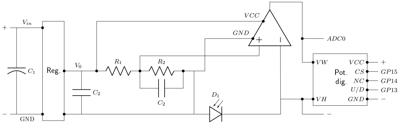
Figura 1: Circuito utilizado para la alimentación del fotodiodo y ajuste de ganancia. Este se compone de un regulador de 3,3 V, un amplificador operacional, el fotodiodo y un potenciómetro digital. El capacitor C_1 es electrolítico de 10\ \mu\text{F} , los capacitores C_2 son capacitores cerámicos de 1\ \text{nF} , ambos se utilizan como filtros. Las resistencias R_1 y R_2 toman valores de 10\ \text{k}\Omega y 220\ \Omega respectivamente. Las salidas CS , NC , U/D del potenciómetro digital controlan el guardado en memoria, el incremento del paso y la dirección de incremento respectivamente. Las conexiones ADC0 , GP hacen referencia a las Raspberry Pi Pico.
