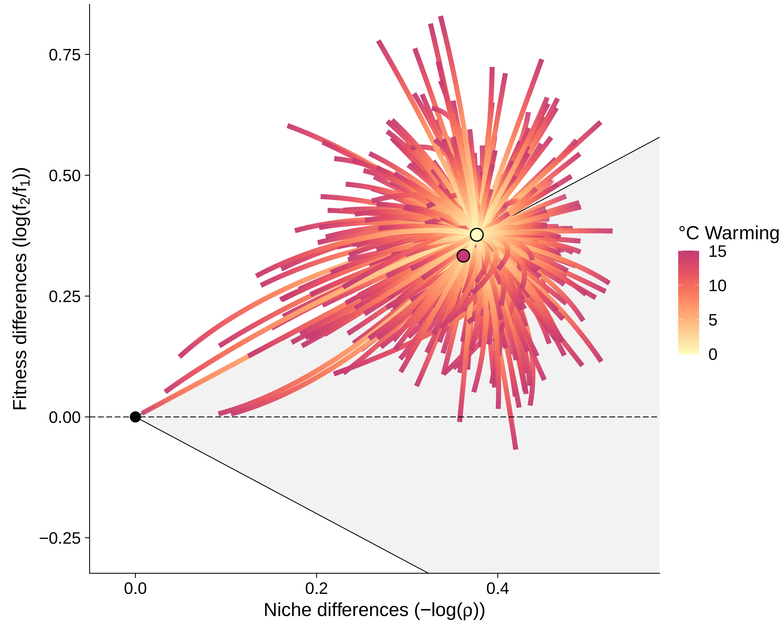
0–15°C Warming
