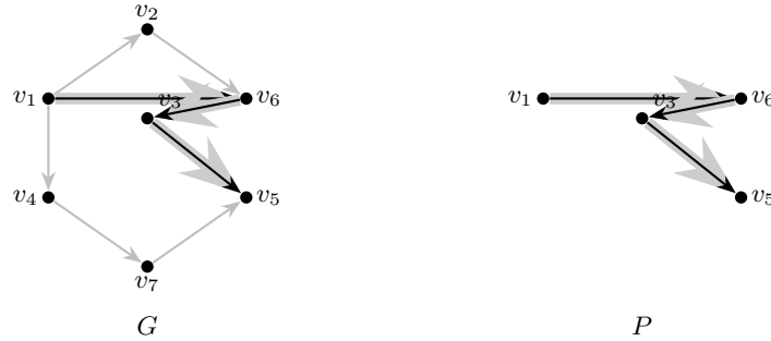
Figura 1.2: Un camino dirigido P = (v_1, v_6, v_3, v_5) en el grafo dirigido G y su representación como subgrafo.
