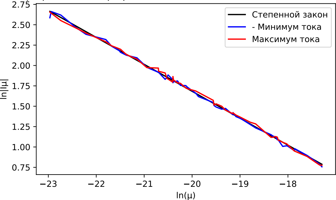
Логарифмический график максимального и минимального тока I_{\mu}(\mu)
