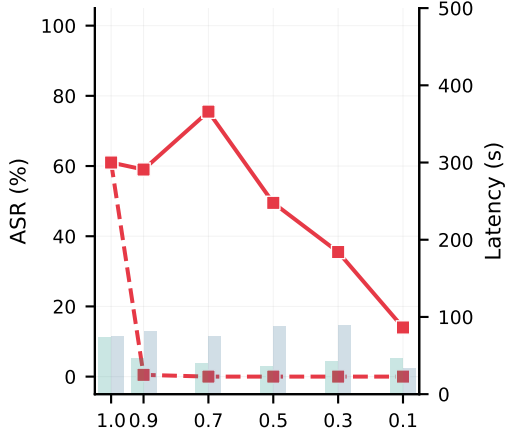
Llama-4-Scout
