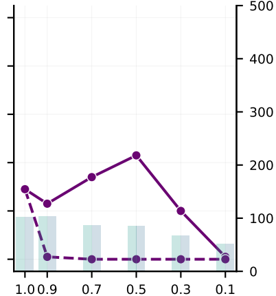
Gemma-2-27B
