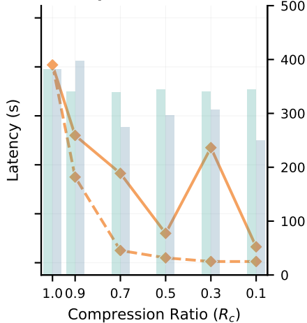
Qwen-1.5-110B
