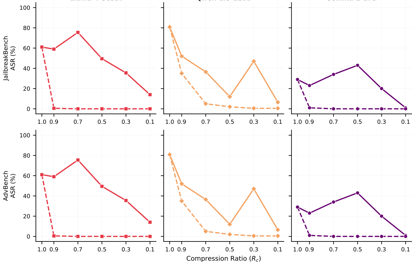
Llama-4-Scout
