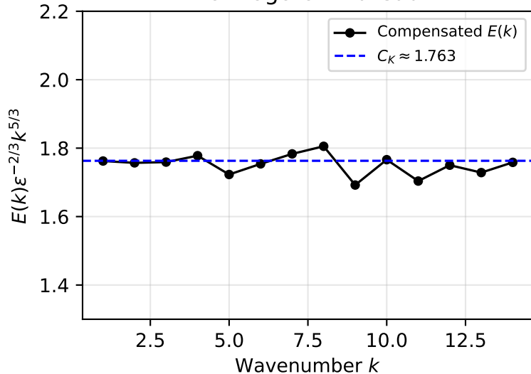
Kolmogorov Plateau
