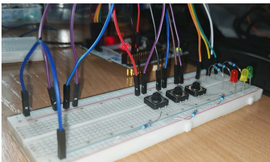
Рисунок 8 – Вид макетной платы
