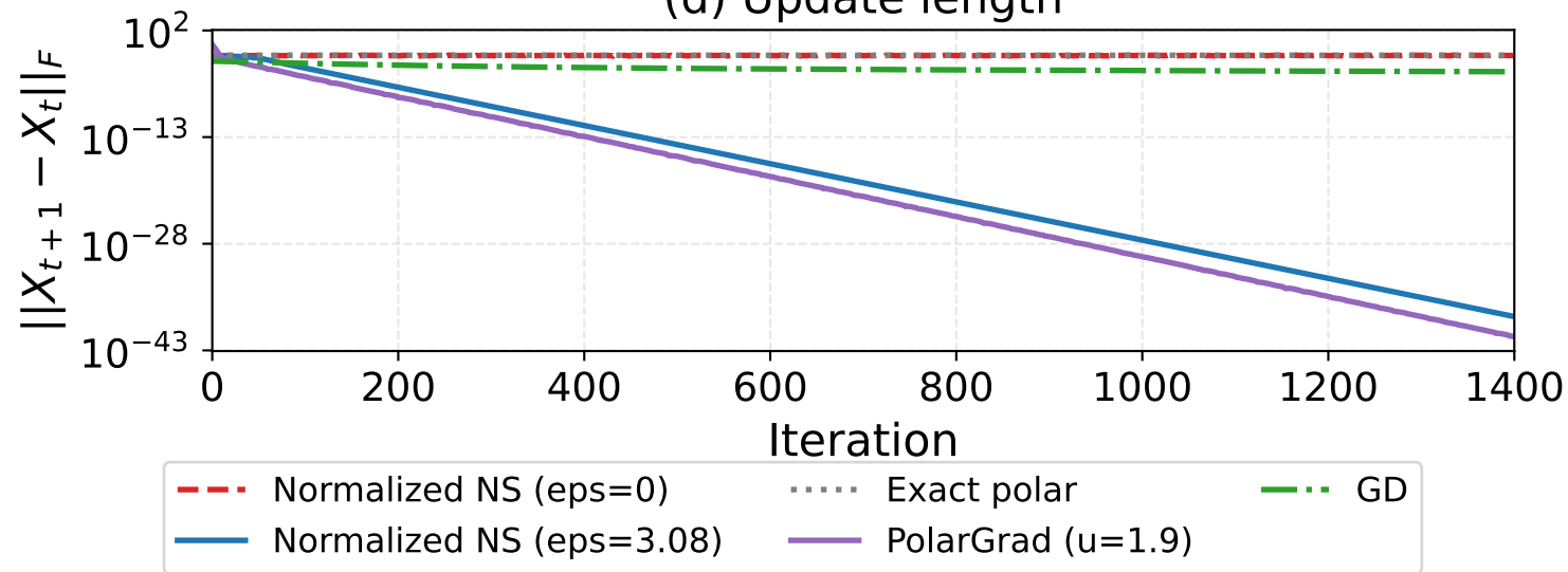
(d) Update length
