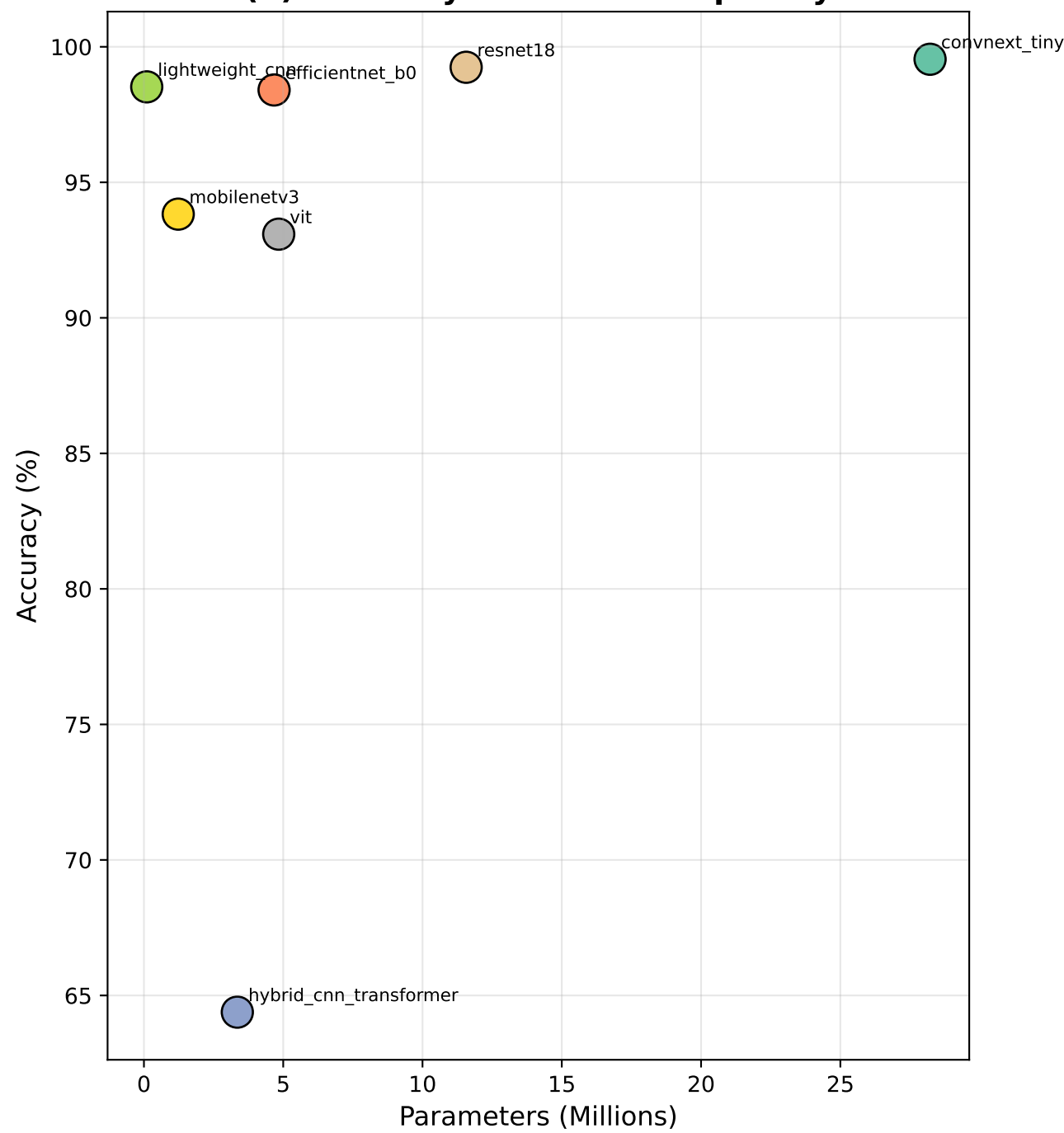
(d) Accuracy vs Model Complexity
