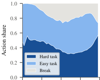
AA-DQN (ours)
