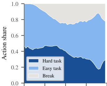
AA-DQN (ours)
