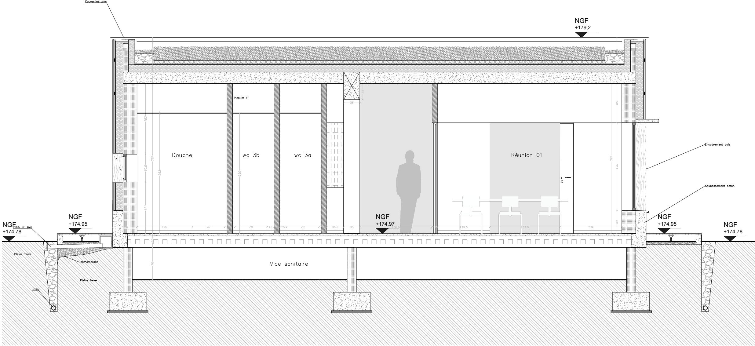
Coupe GG' – 1/100
