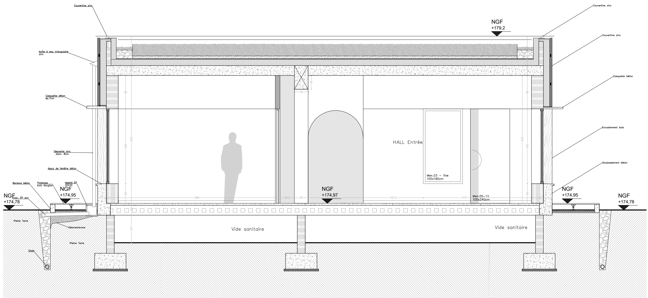
Coupe CC' – 1/100
