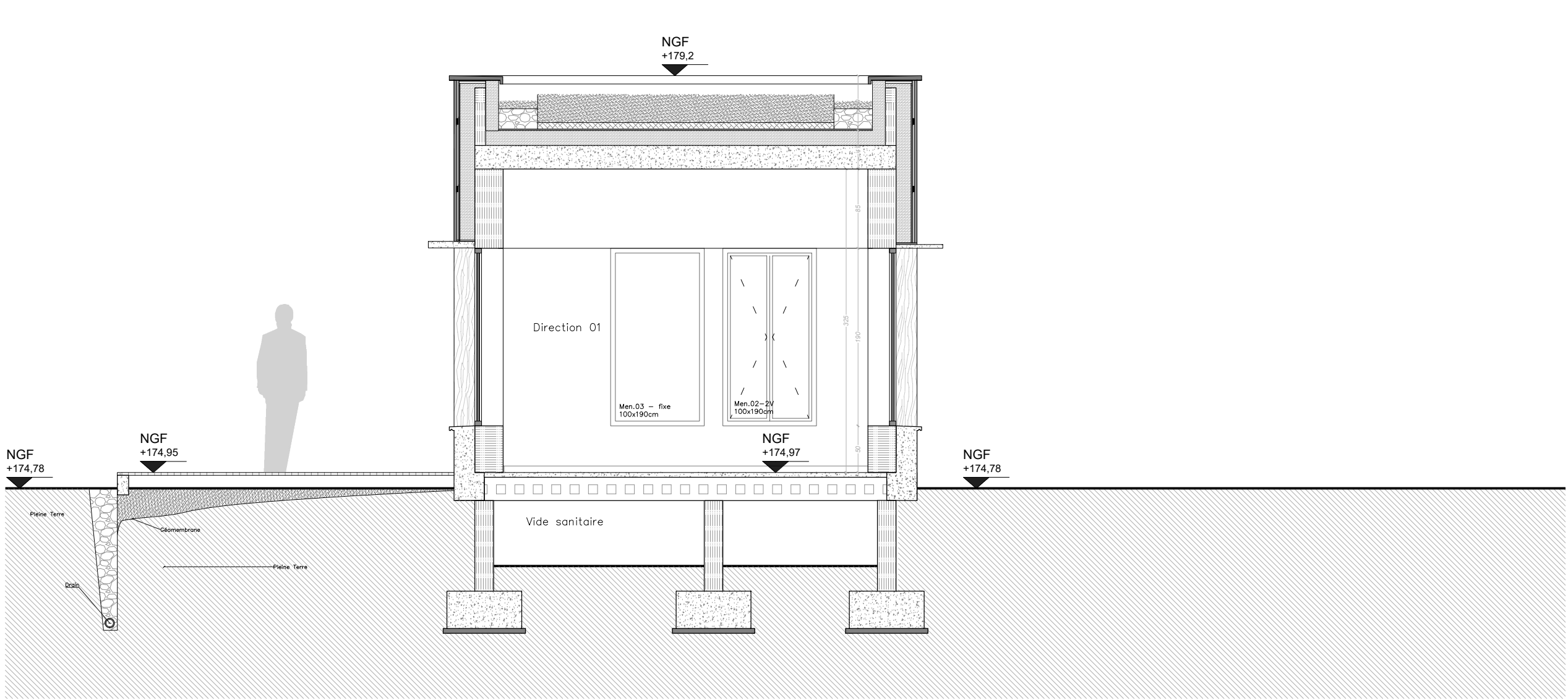
Coupe AA' – 1/100
