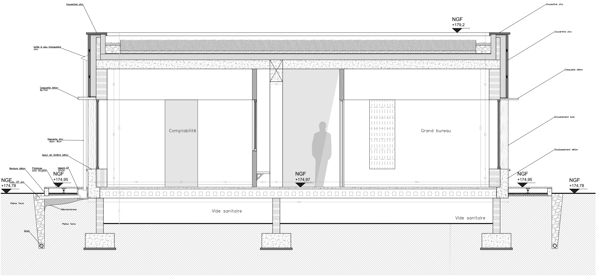
Coupe DD' – 1/100
