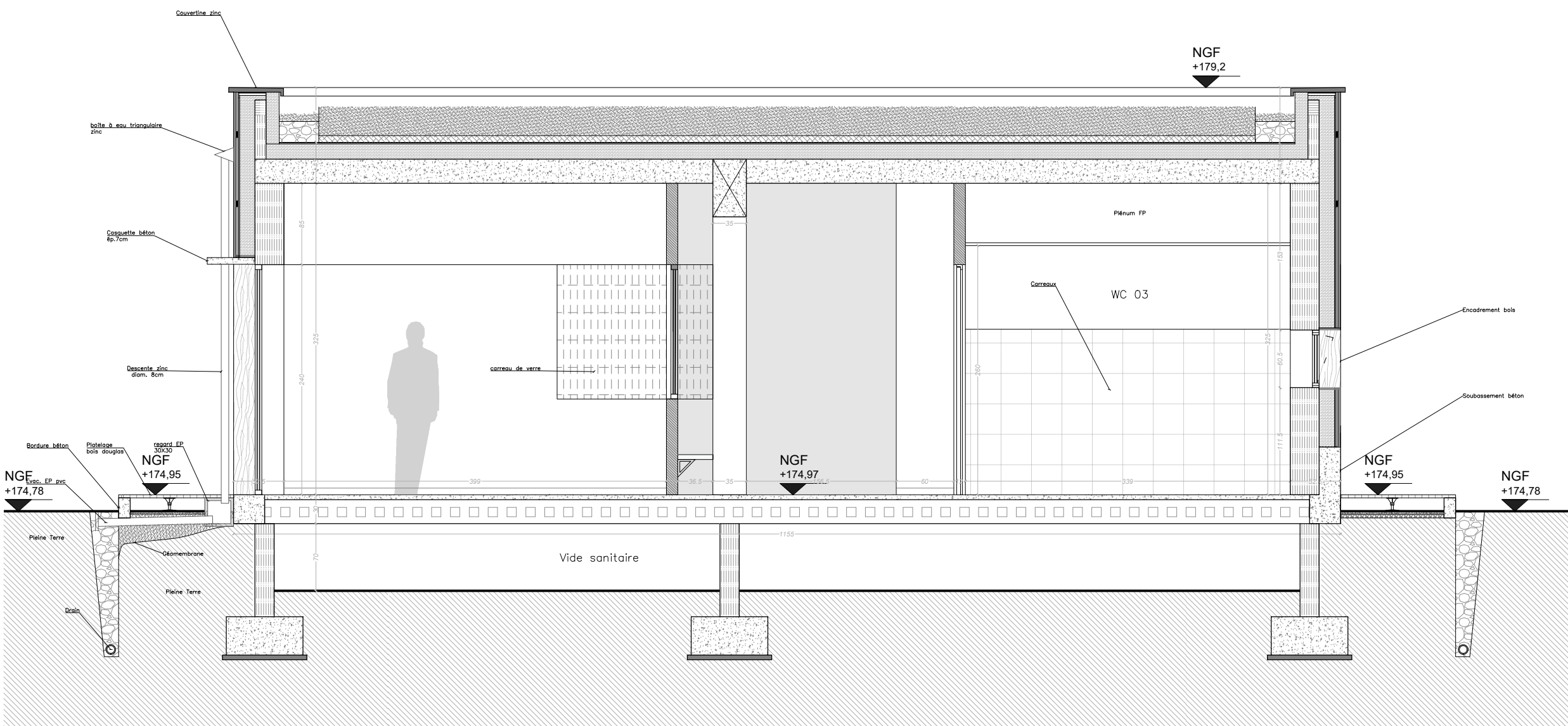
Coupe EE' – 1/100
