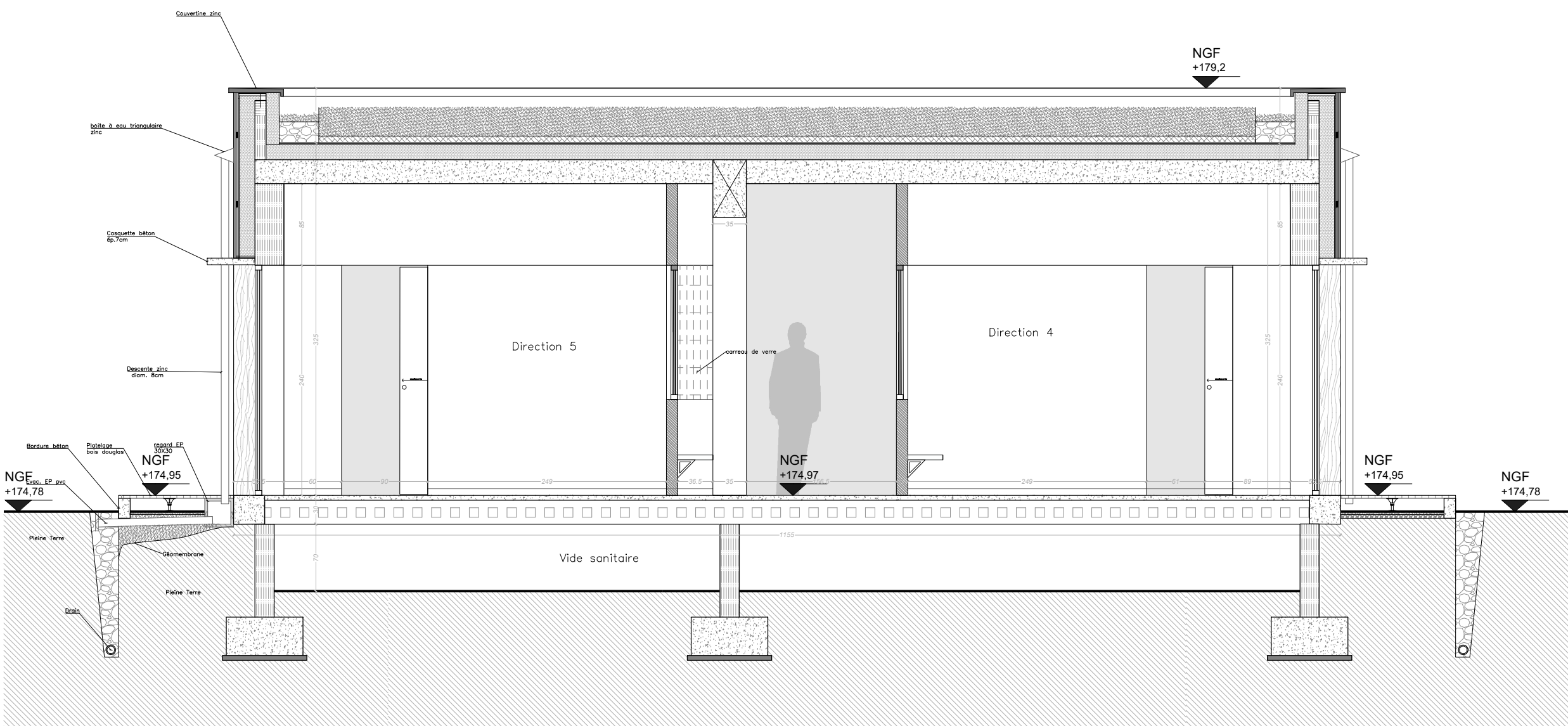
Coupe FF' – 1/100
