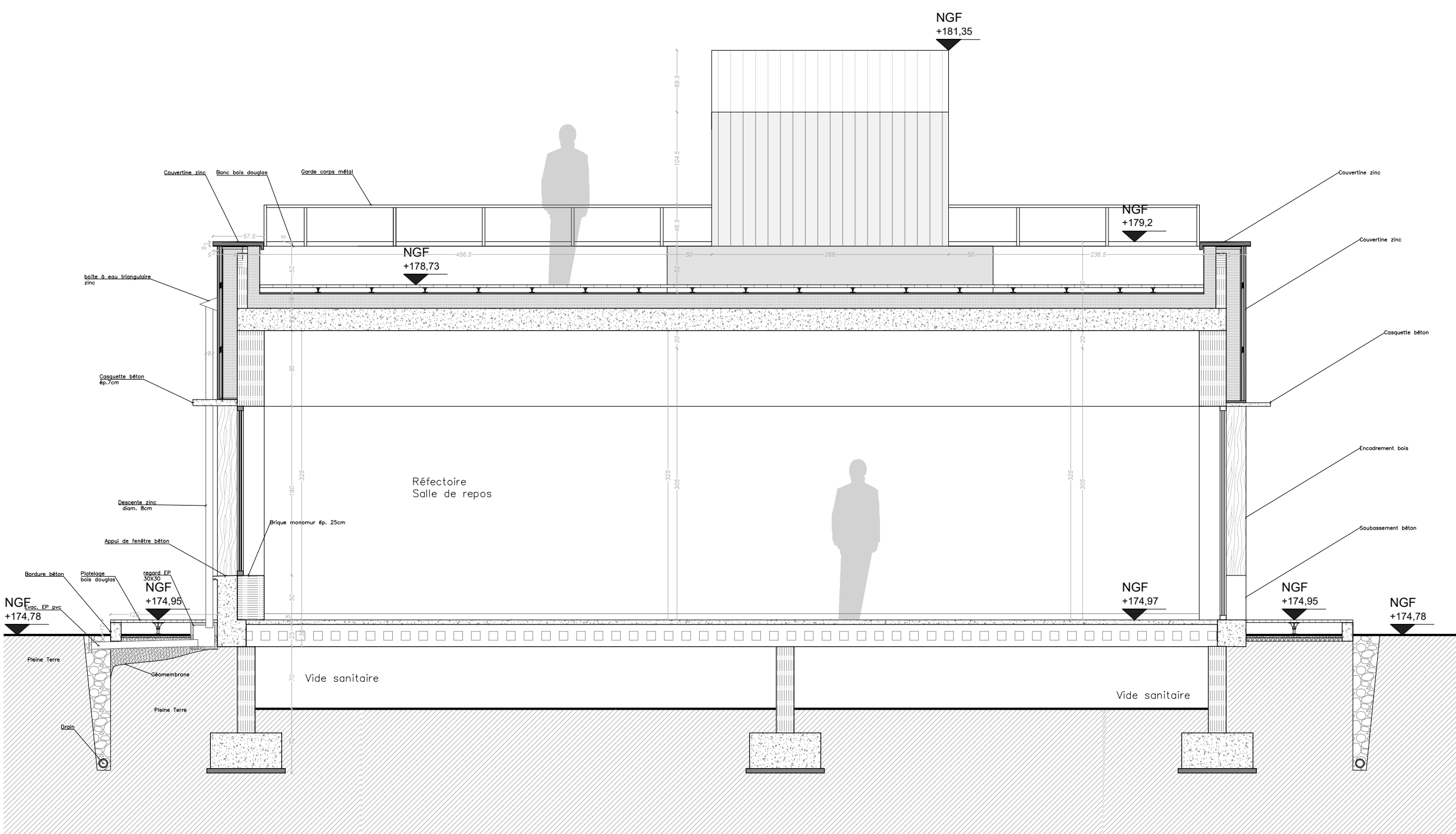
Coupe ii' – 1/100
