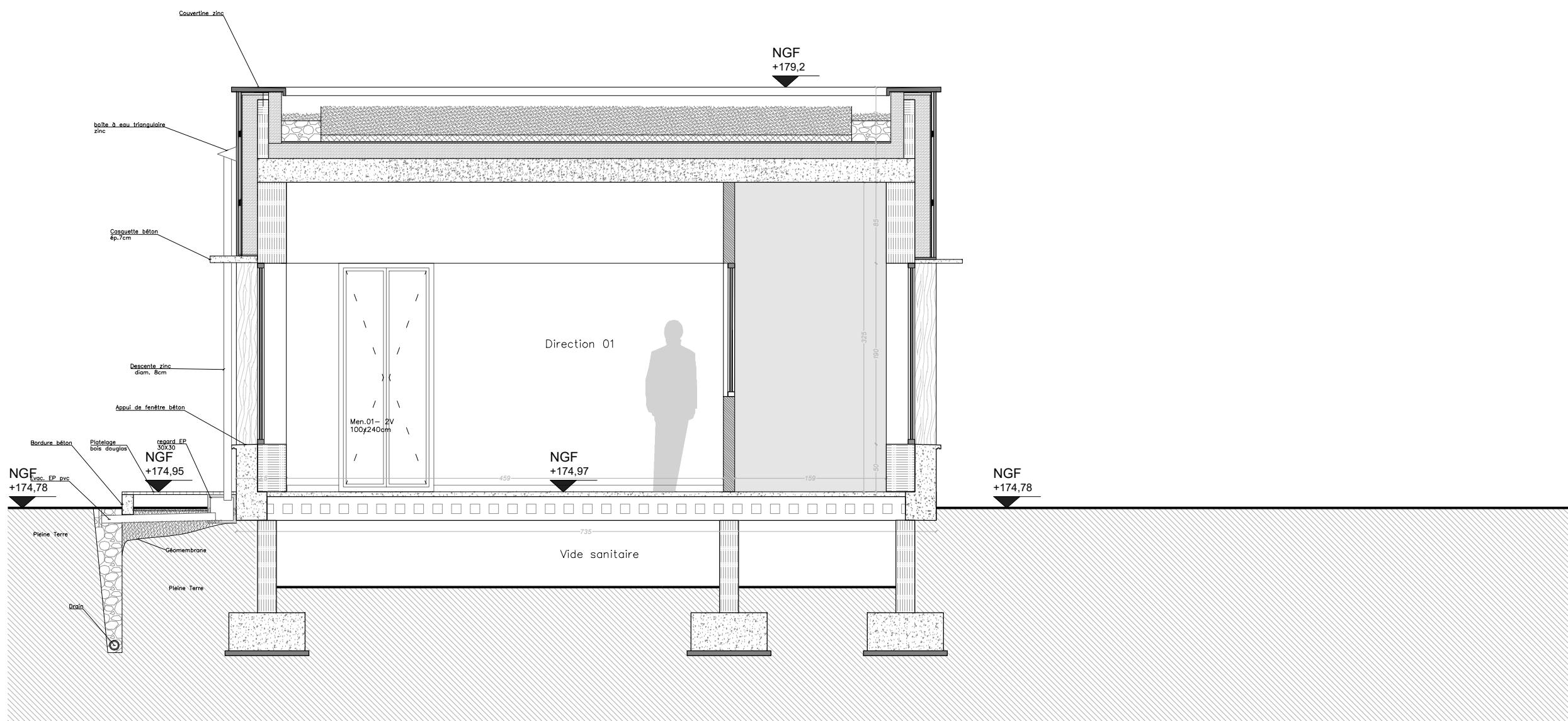
Coupe BB' – 1/100
