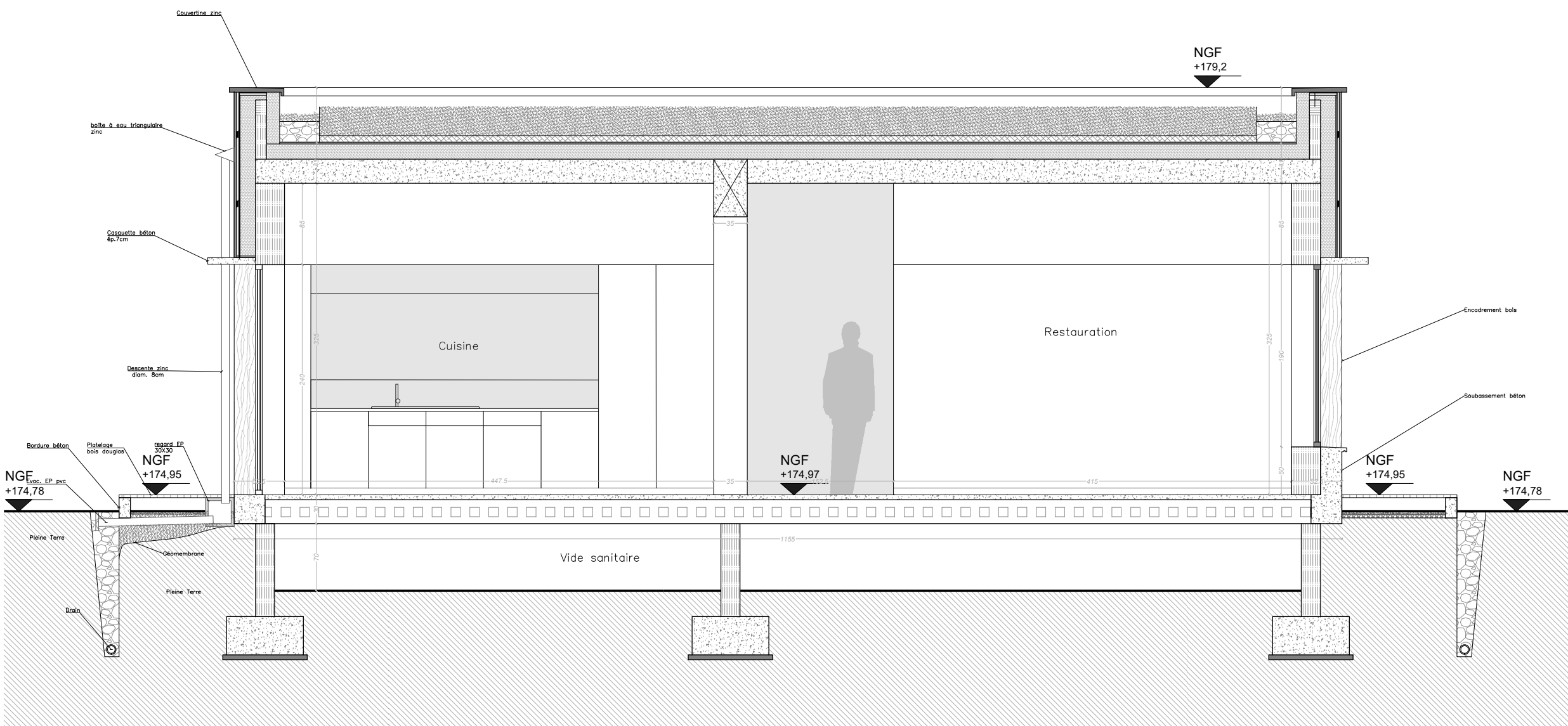
Coupe HH' – 1/100
