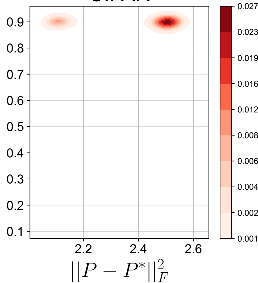
CIFAR
