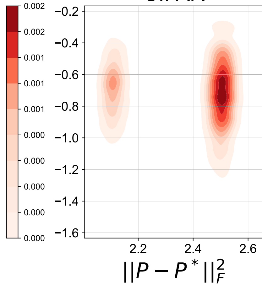
CIFAR
