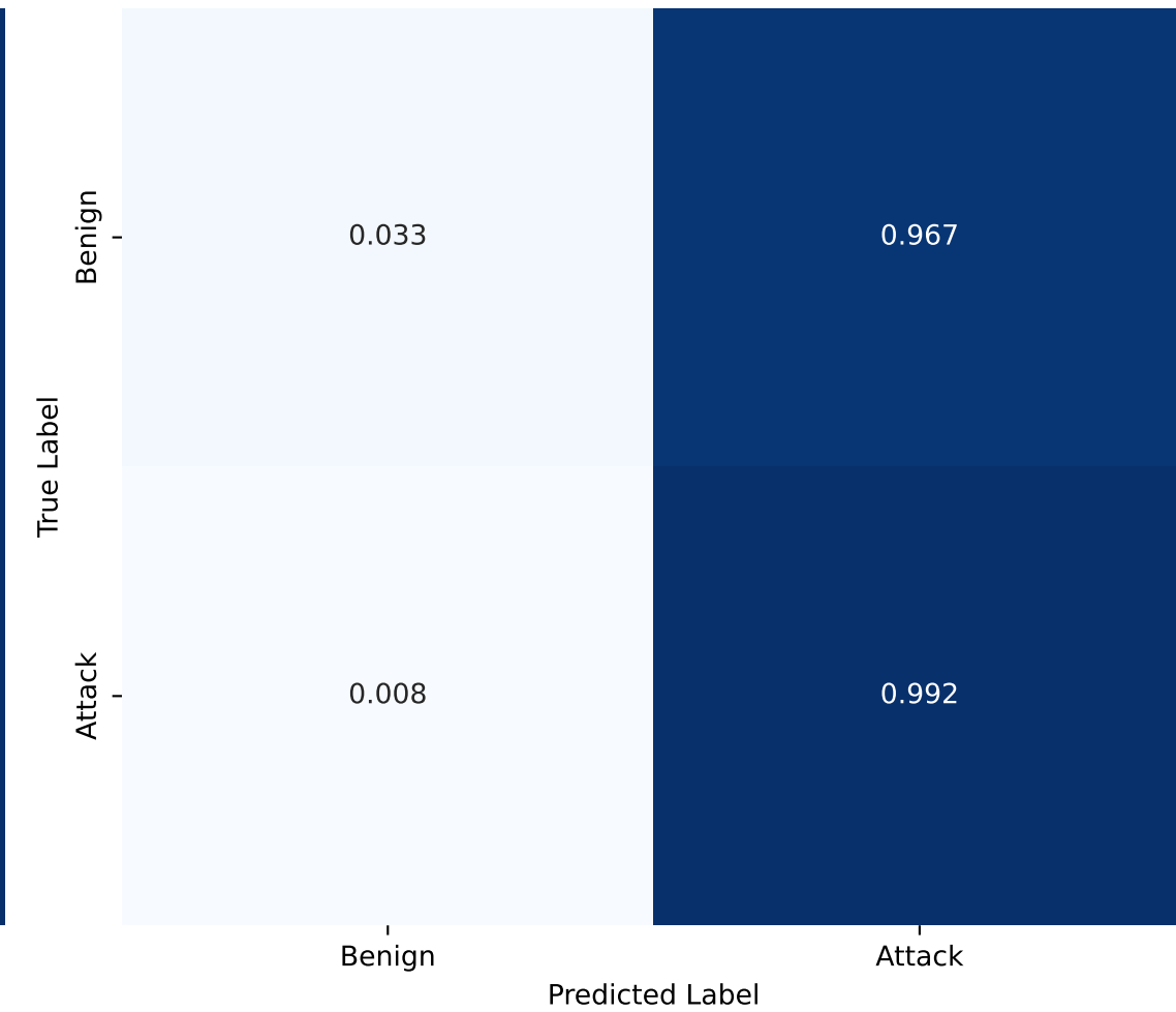
D1 -&gt; D3 DANN (Calibrated)
