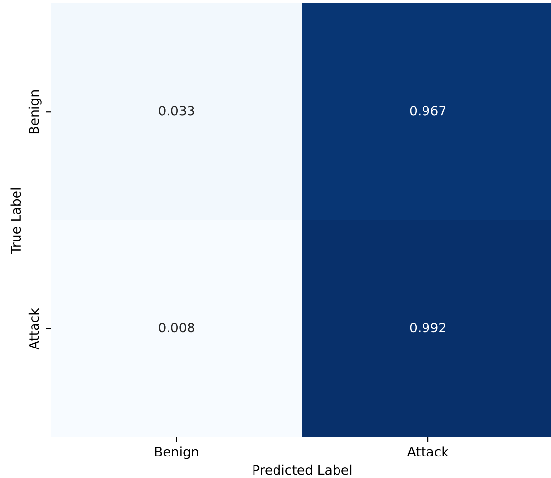
D1 -&gt; D3 Baseline (Calibrated)
