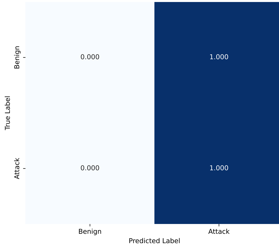
D1 -&gt; D3 CORAL (Calibrated - BEST)
