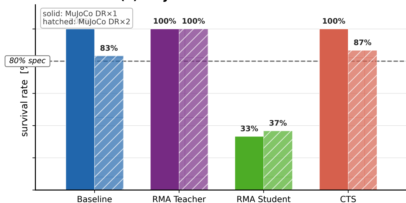
(D) Sim2Sim @ DR \times 2: Isaac vs MuJoCo (worst-case)
