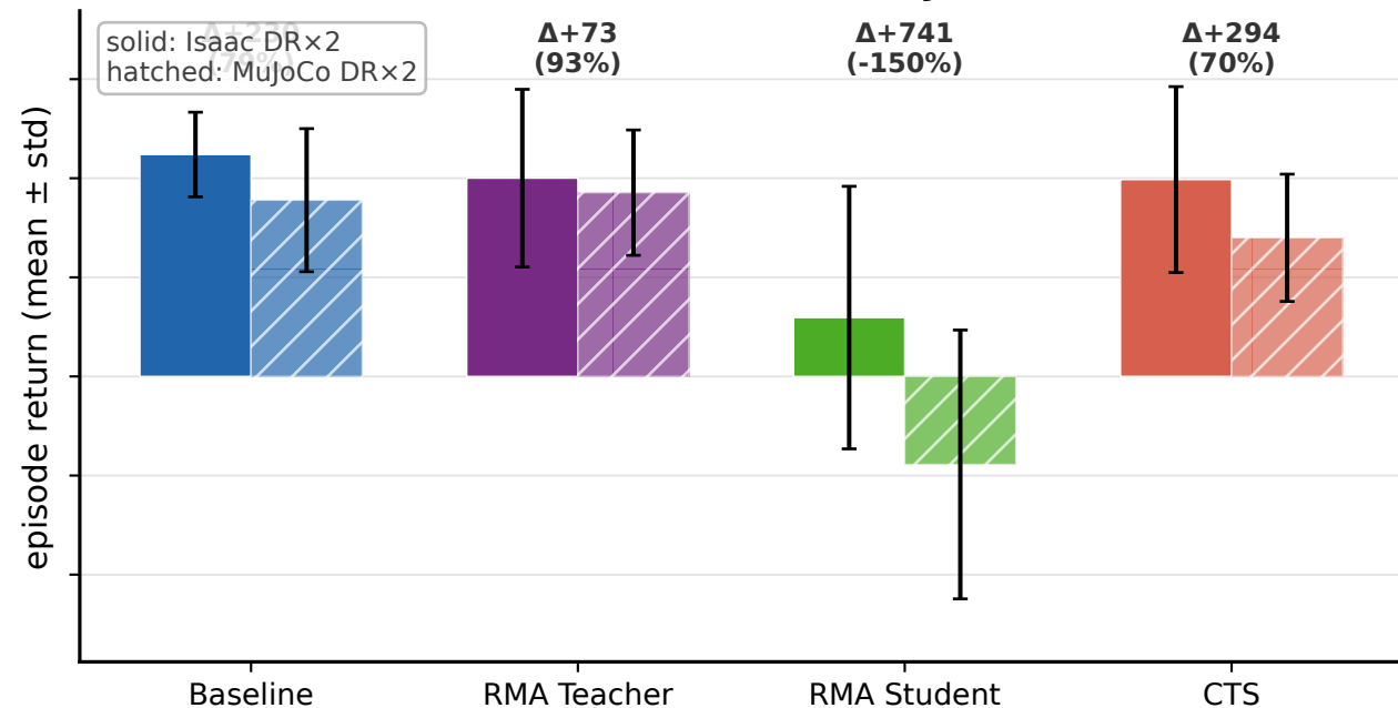
(D) Sim2Sim @ DR×2: Isaac vs MuJoCo (worst-case)
