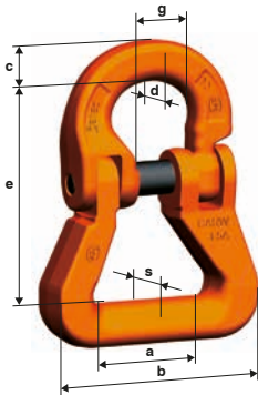
CARW Elo de ligação para cintas textéis
