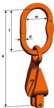
VVKW 1 Elo de suspensão com acoplamento
