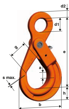
LHW Gancho olhal autoblocante
