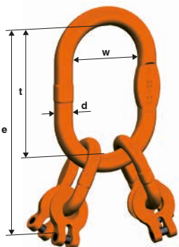
KAGW 4 Elo de suspensão com acoplamento
