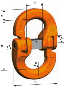
CLW Connex Elo de ligação
