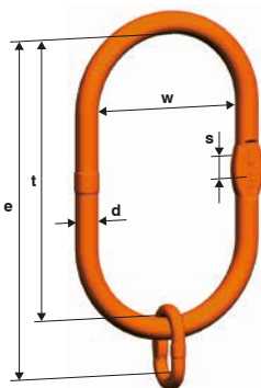
VLW 1 Elo especial de 4 ramais
