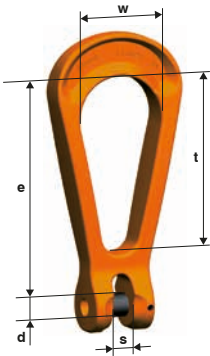
KOW Elo de suspensão com acoplamento
