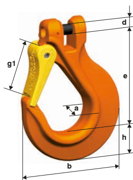
BKHSW Gancho clevis com trava extra grande e acoplamento
