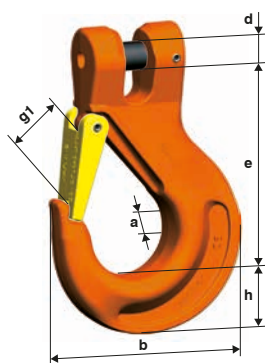
KHSW Gancho clevis com trava e acoplamento
