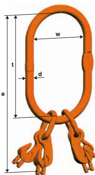
LXKW 4 Elo de suspensão com acoplamento
