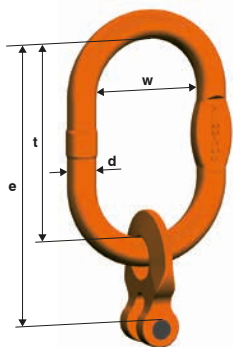
KAGW 1 Elo de suspensão com acoplamento
