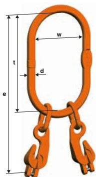
LKXW 2 Elo de suspensão com acoplamento
