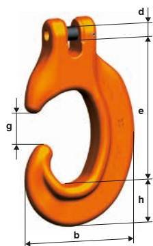
KCHW Gancho em C com acoplamento
