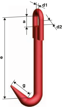
BA Gancho para fardos
