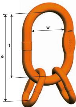
VW Elo de Suspensão de 3 e 4 ramais
