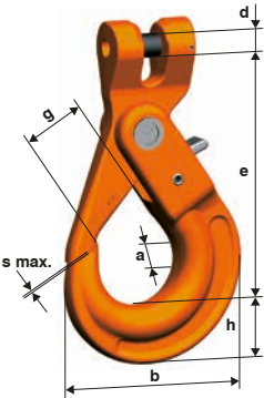
KLHW Gancho clevis autoblocante
