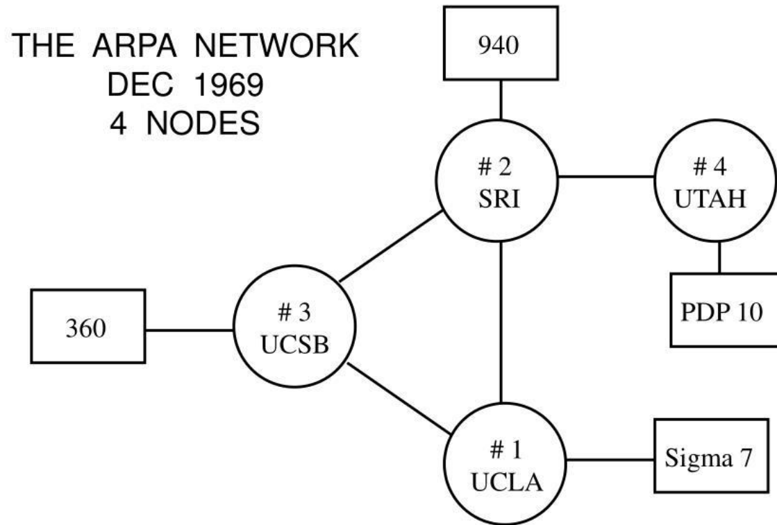
図 1. 1 ARPAネットの構成図(1969)
