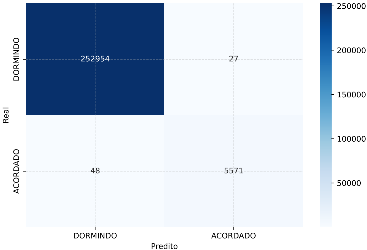
Matriz de Confusão - LSTM
