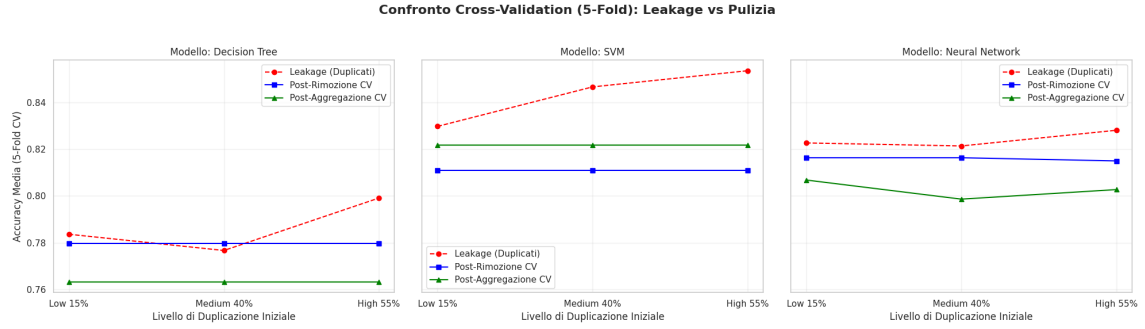
Figura 44: Confronto tra le strategie di gestione dei duplicati in Cross-Validation per i tre modelli analizzati.
