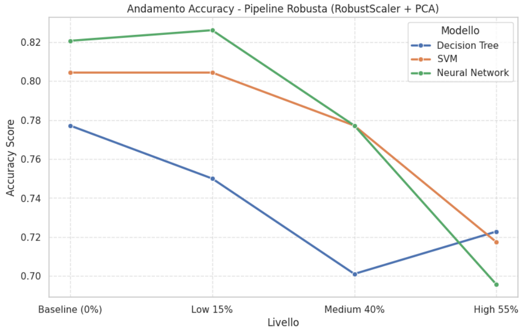
Figura 45: Andamento dell'Accuracy con pipeline robusta applicata al rumore gaussiano e di swap.
