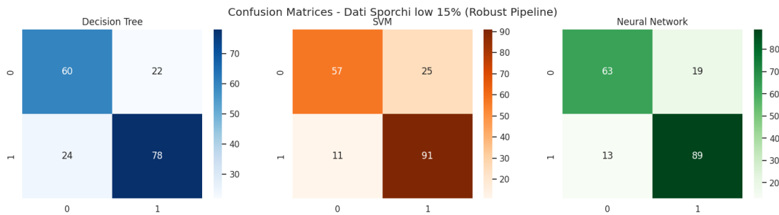
Figura 47: Matrici di confusione dei modelli con pipeline robusta al 15% di rumore (gaussiano e swap).
