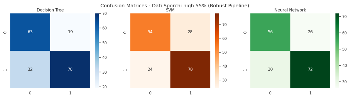
Figura 49: Matrici di confusione dei modelli con pipeline robusta al 55% di rumore (gaussiano e swap). Si noti l'elevato numero di falsi negativi nel Decision Tree.
