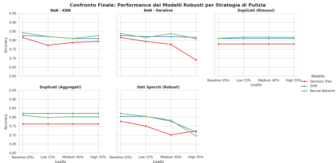
Figura 51: Confronto finale delle prestazioni dei modelli robusti per strategia di pulizia dei dati
