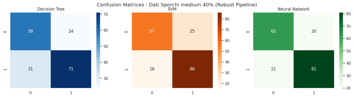
Figura 48: Matrici di confusione dei modelli con pipeline robusta al 40% di rumore (gaussiano e swap).
