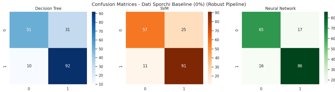
Figura 46: Matrici di confusione dei modelli con pipeline robusta sui dati originali (Baseline 0%).
