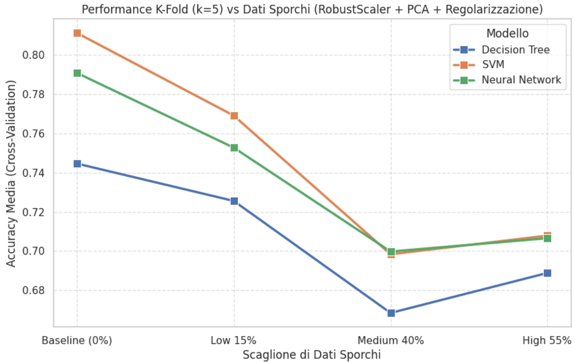
Figura 50: Andamento dell'Accuracy media in Cross-Validation (K=5) per i modelli addestrati con pipeline robusta al variare del rumore gaussiano e di swap.
